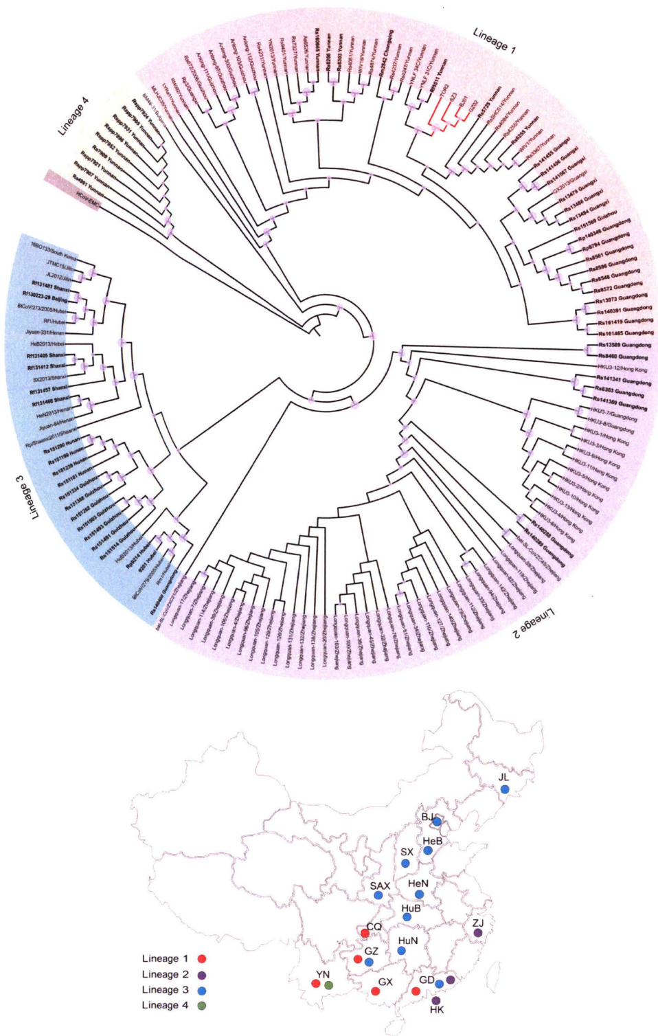
图 3.1 基于完整的 RdRp 序列的 SARS 样冠状病毒和 SARS 冠状病毒的系统进化分析。
