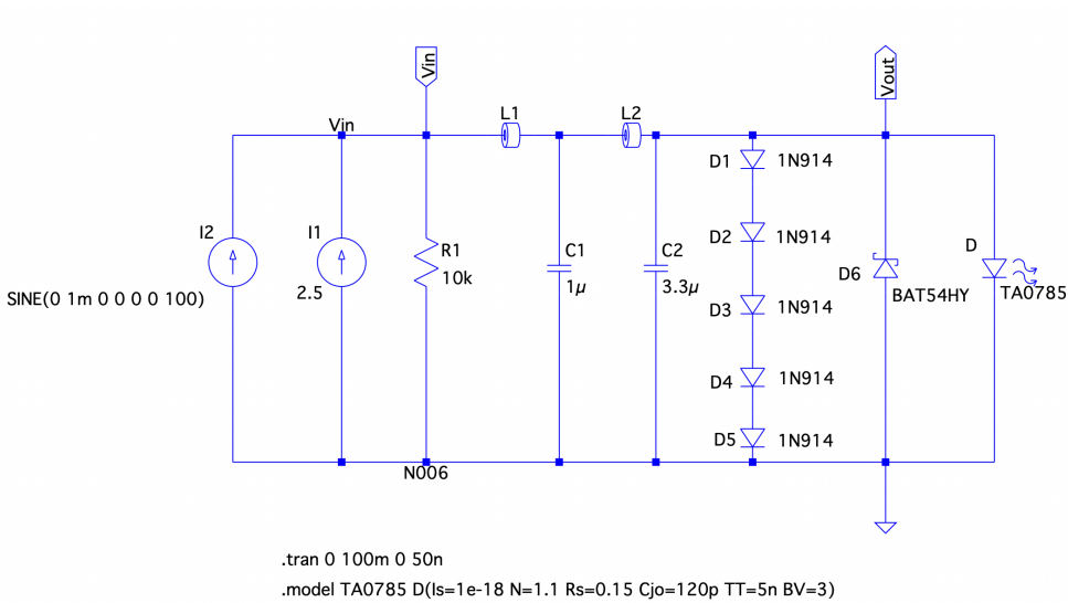
Figure 1: Simulación circuito de protección del TA
