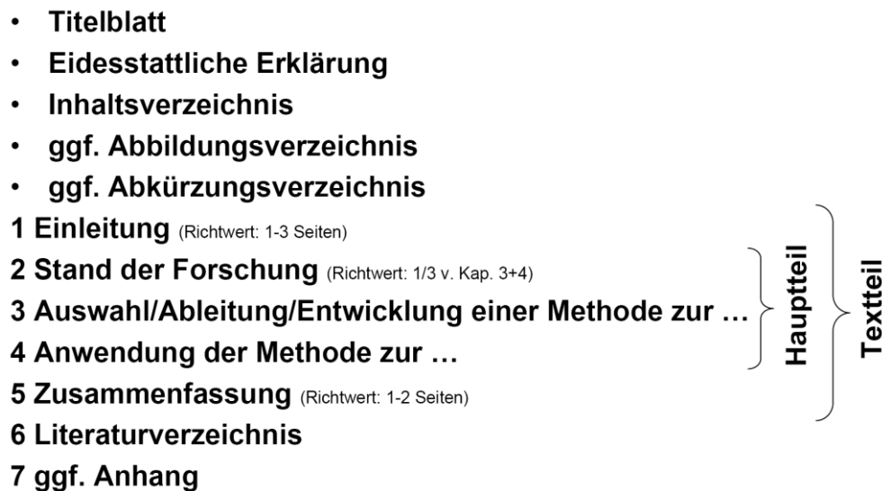
Abbildung 1: Gliederungsgerüst
