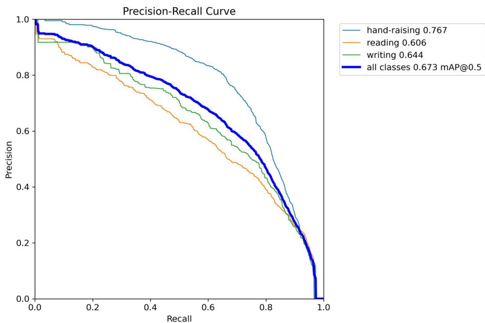
YOLO26s - PR curve
