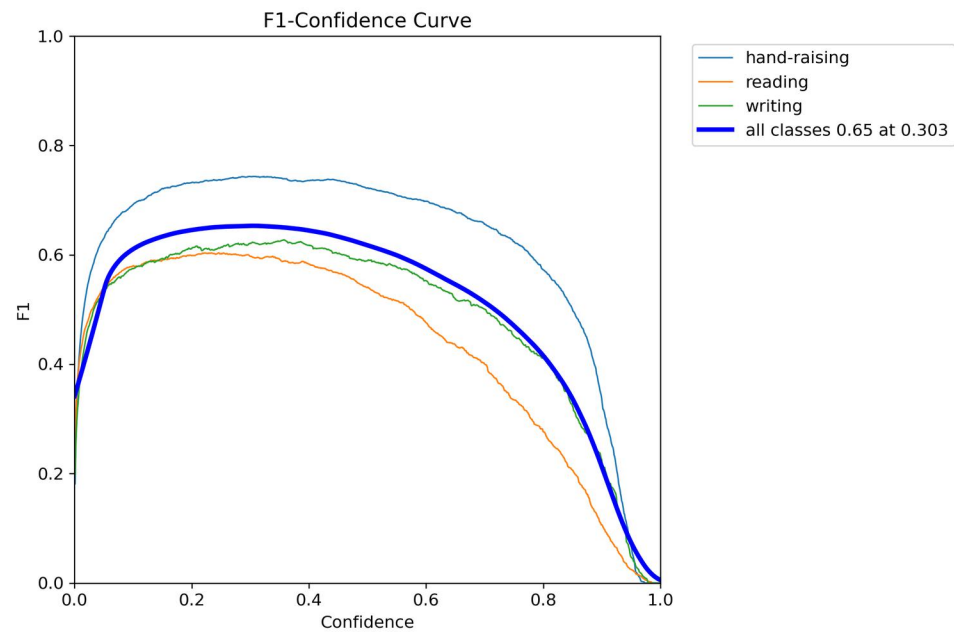
BAC-SSM-YOLO - F1 curve
