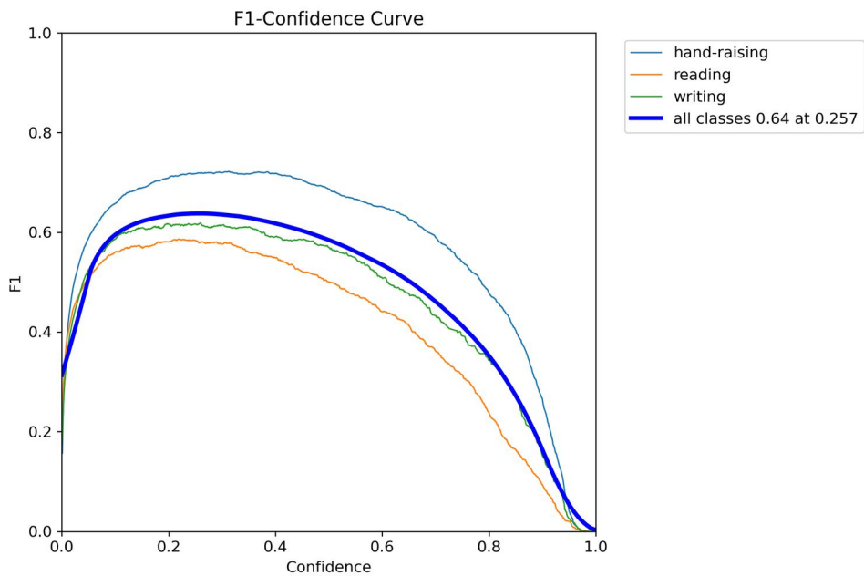
YOLO26s - F1 curve
