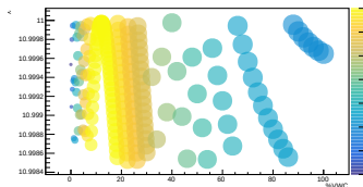
LCO_event_157_timegrid_15_ndet_11_scatterplo
