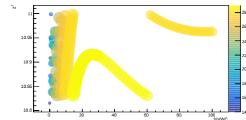
LCO_event_159_timegrid_15_ndet_11_scatterplo
