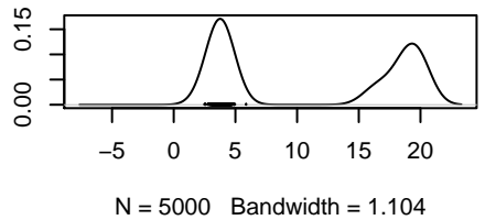
Density of par 2
