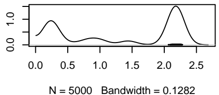
Density of par 4
