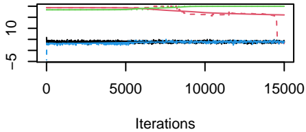
Trace of par 2
