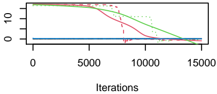
Trace of par 1
