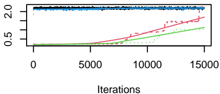
Trace of par 4
