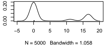
Density of par 1
