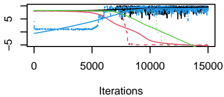
Trace of par 3
