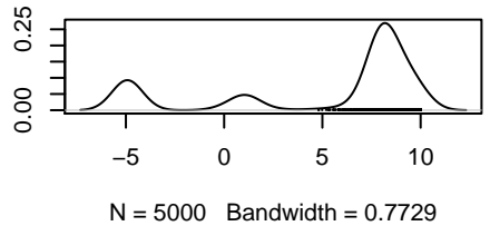
Density of par 3
