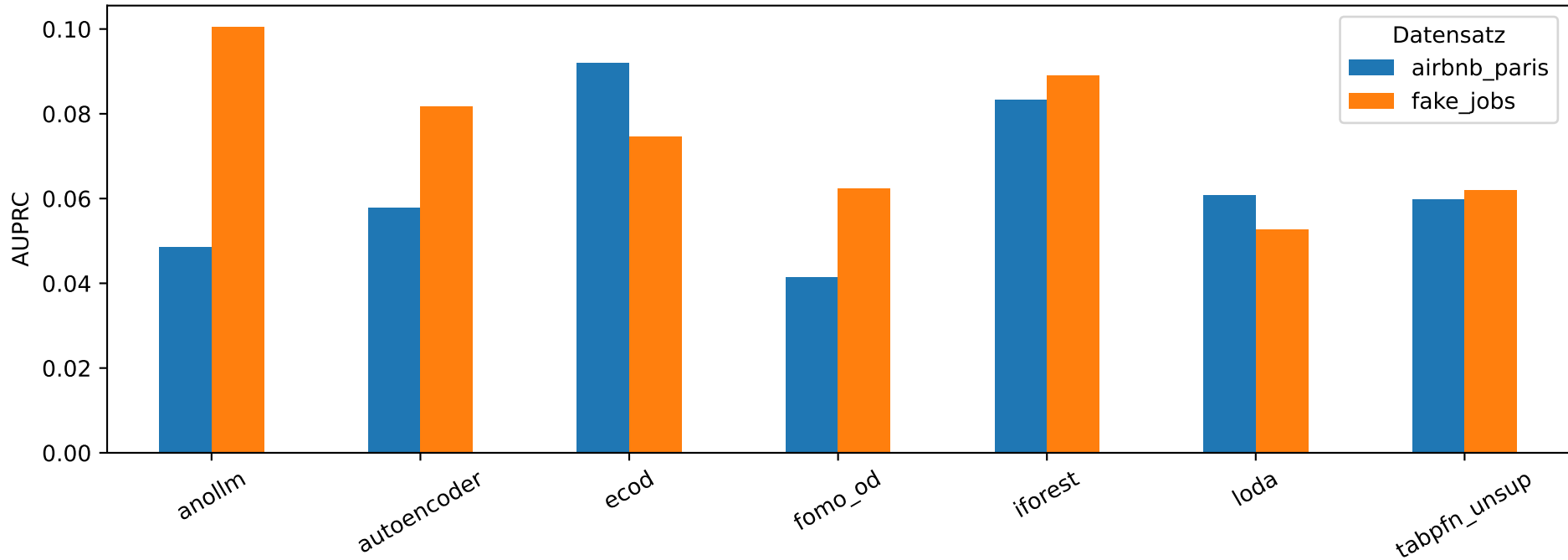
Experiment 1 - AUPRC (beide Datensätze)
