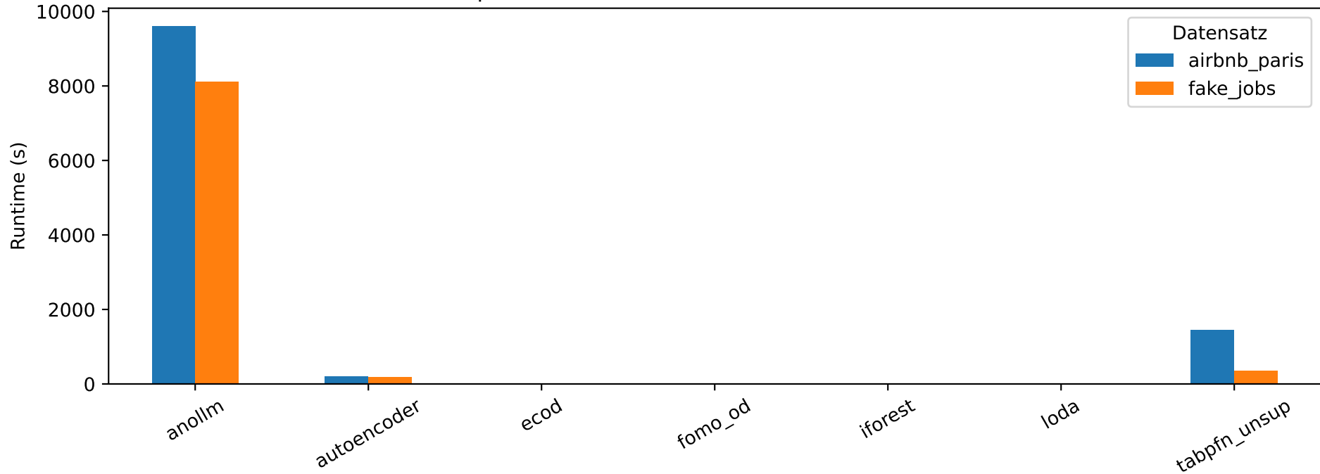
Experiment 1 - Runtime (s) (beide Datensätze)
