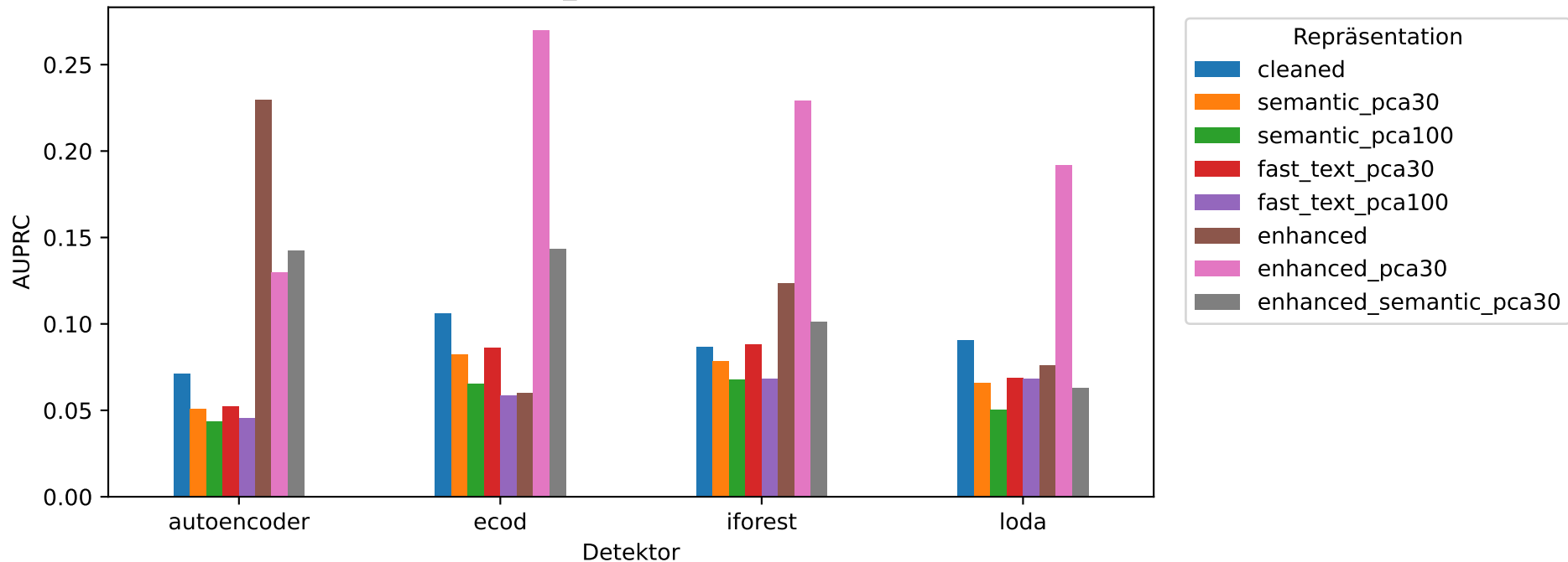
Experiment 2 - airbnb_paris: AUPRC je Repräsentation
