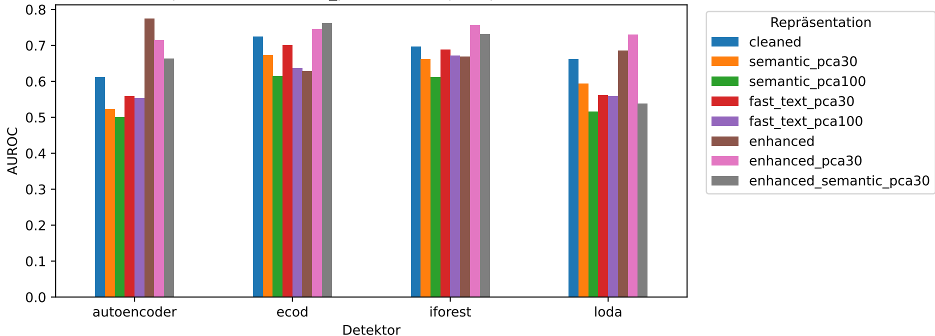
Experiment 2 - airbnb_paris: AUROC je Repräsentation
