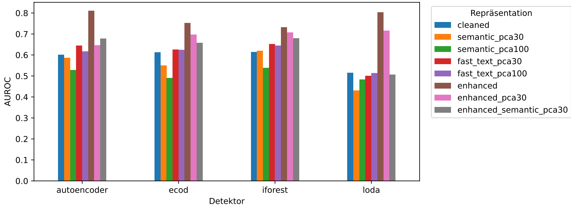
Experiment 2 - fake_jobs: AUROC je Repräsentation
