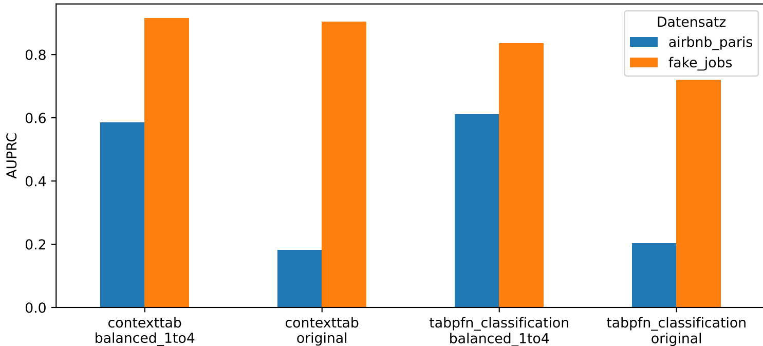
Experiment 4 - AUPRC (beide Datensätze)
