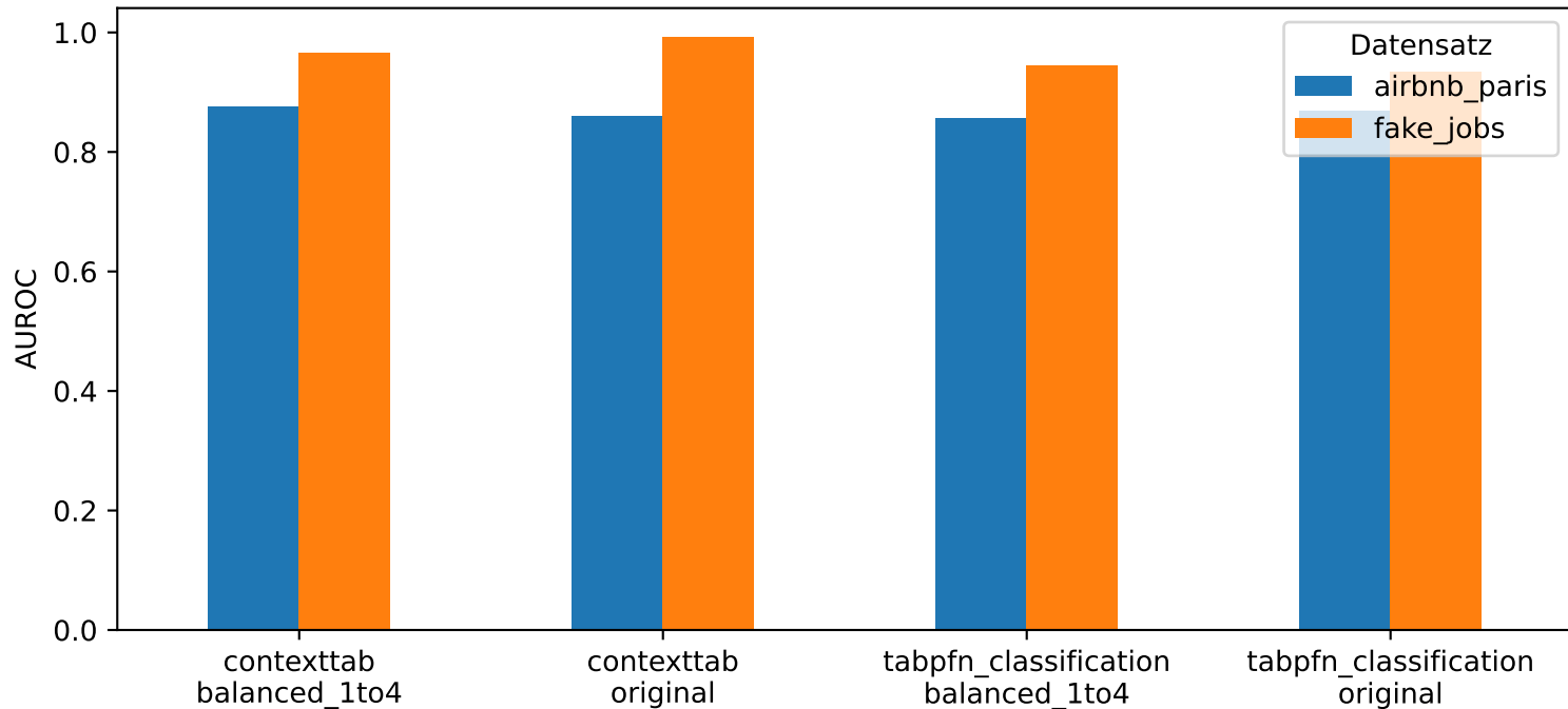
Experiment 4 - AUROC (beide Datensätze)
