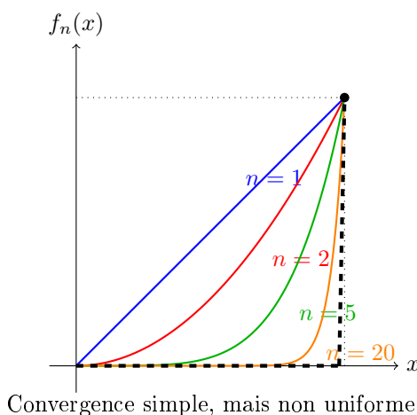
FIGURE 1 – Suite de fonctions f_n(x) = x^n sur [0, 1] convergeant vers la fonction limite discontinue.
