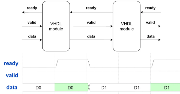
Figura 2.4: Handshake básico del protocolo AXI. Fuente: [Jen22]
