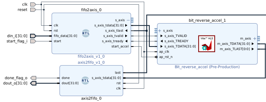
Figura 4.1: Digrama de bloques en Vivado
