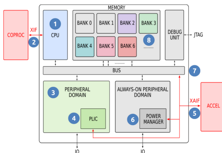
Figura 4.4: Arquitectura de GR-HEEP integrando un acelerador (5) Fuente: [Qui25a]
