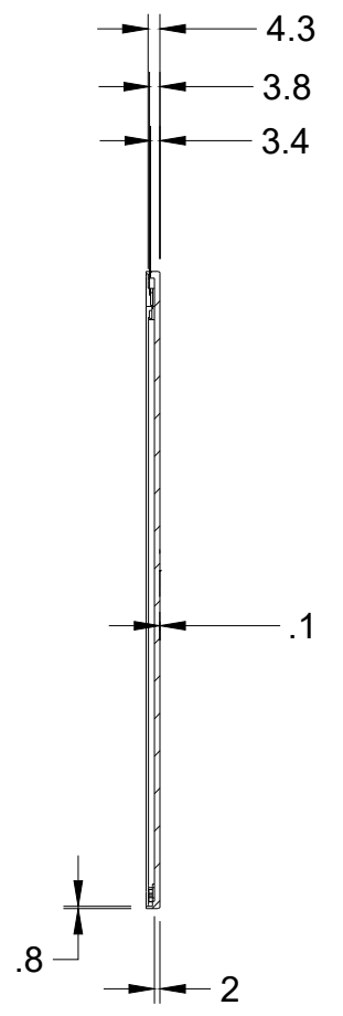
SECTION A-A
