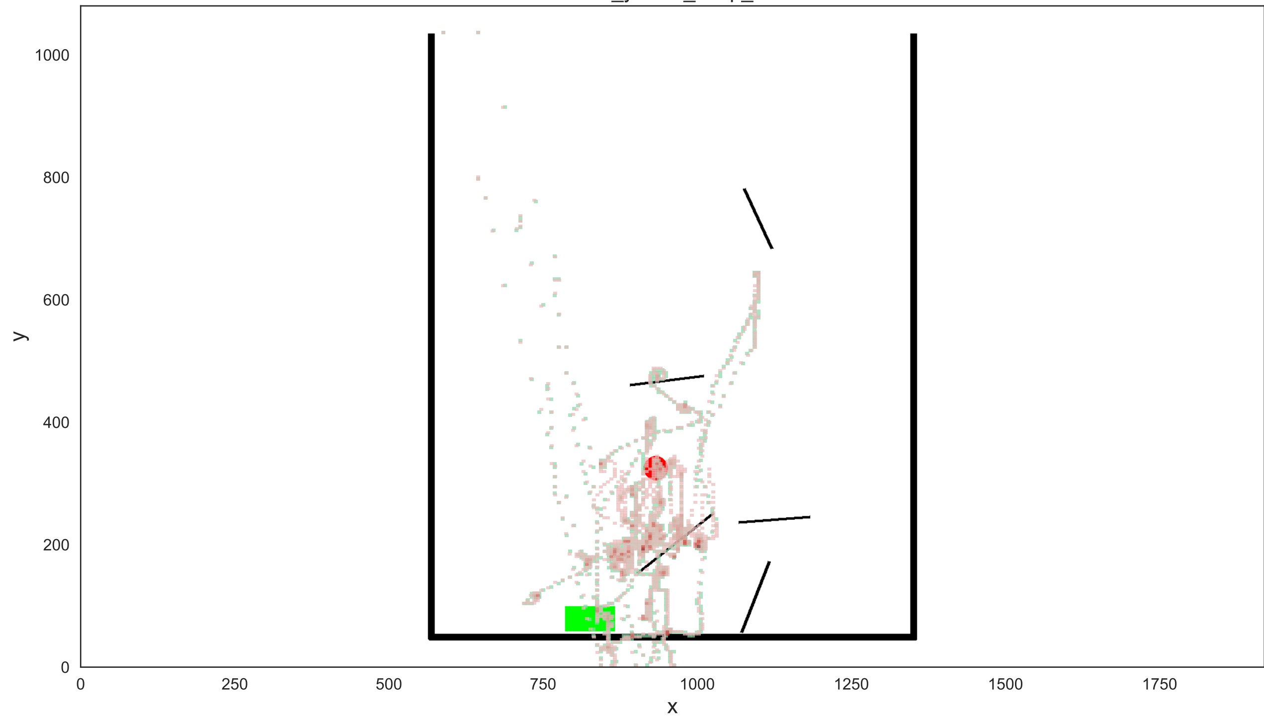
low_yescol_nosp_3
