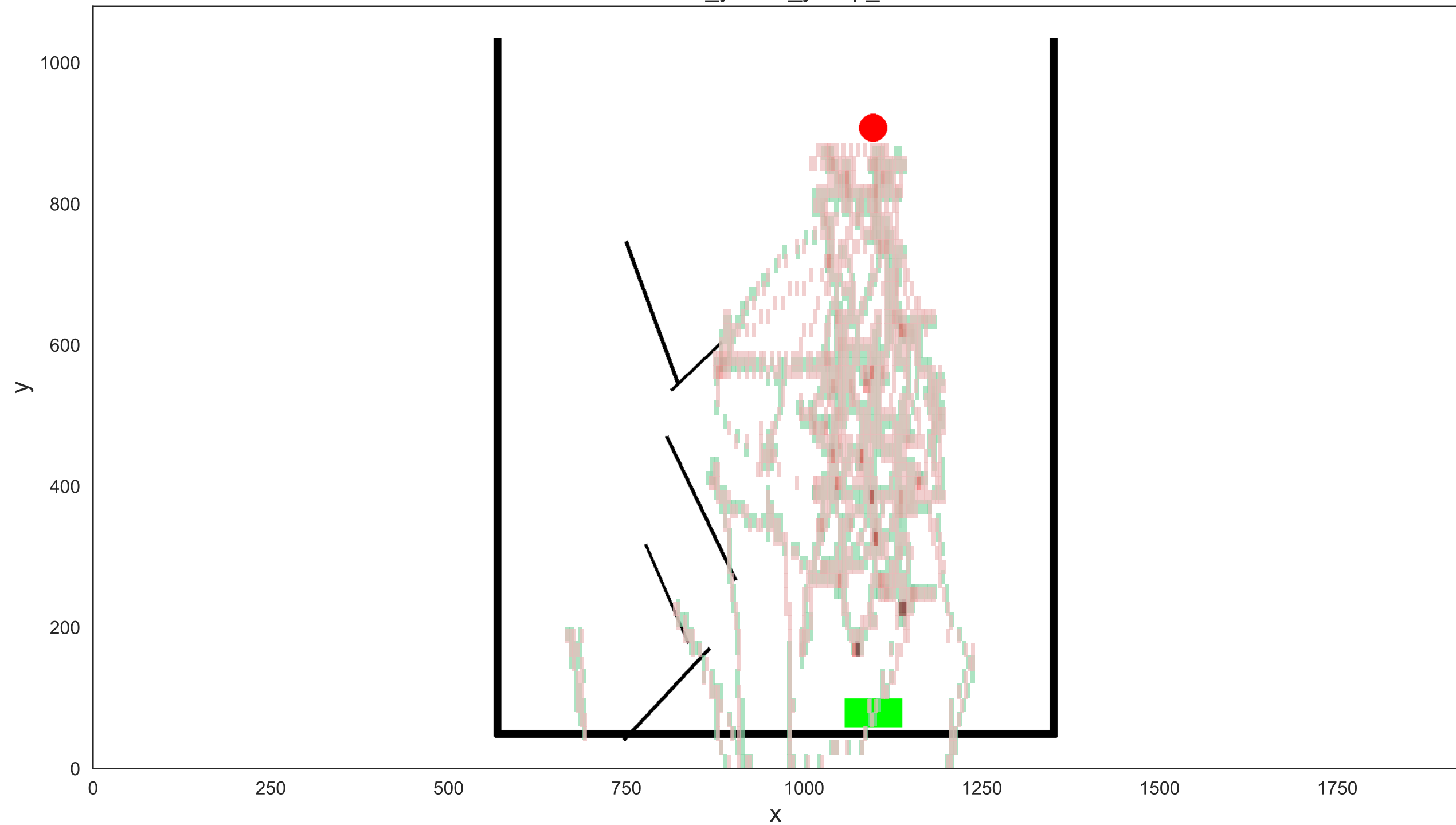
med_yescol_yessp_3
