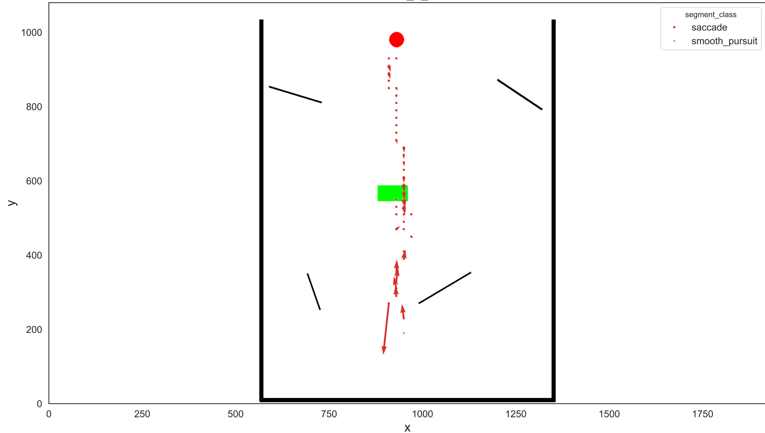
scene_2_13
