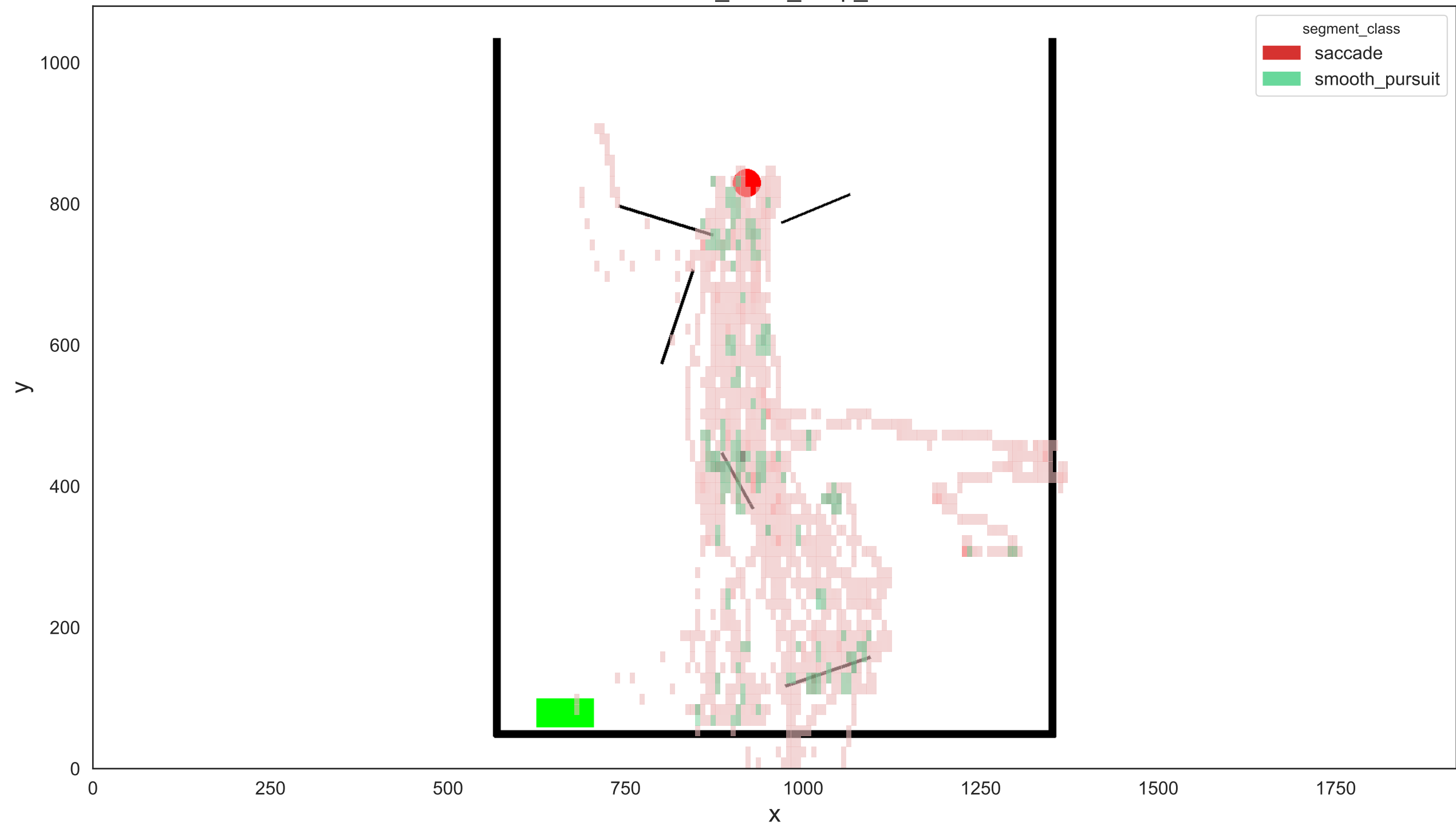
med_nocol_nosp_4
