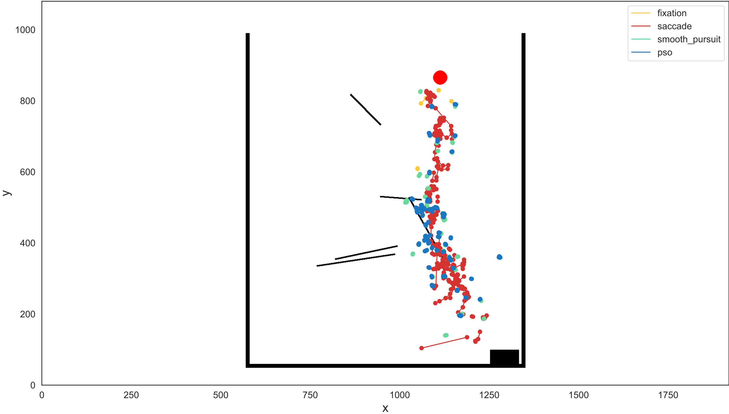
Scene: med_yescol_nosp_1
