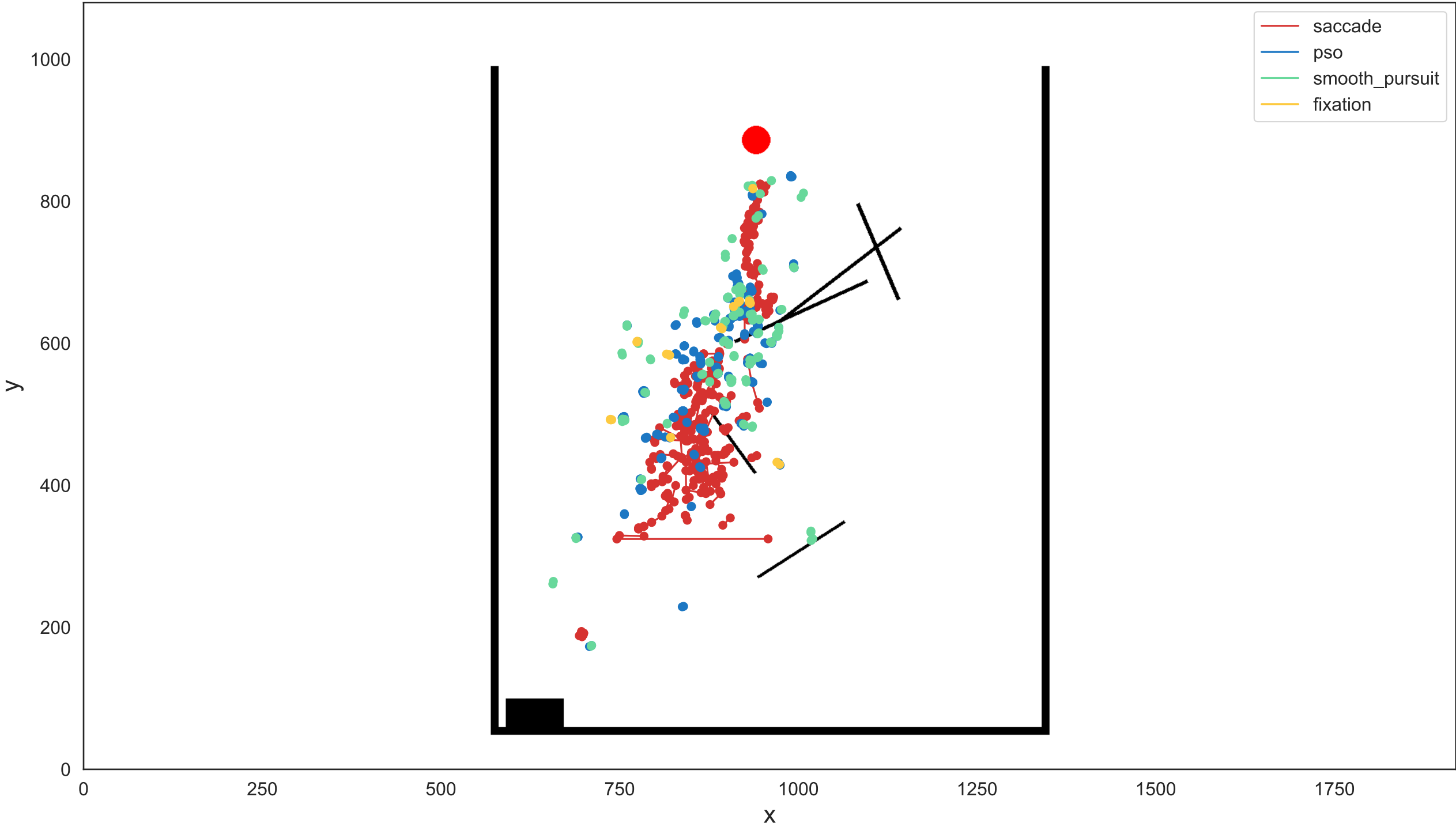
Scene: med_yescol_nosp_4
