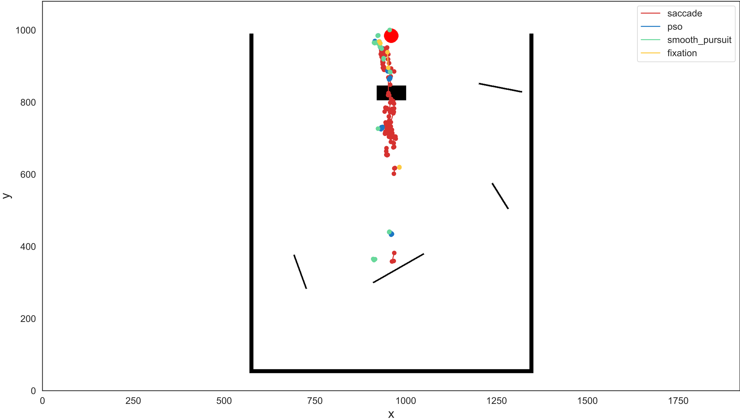
Scene: scene_1_1
