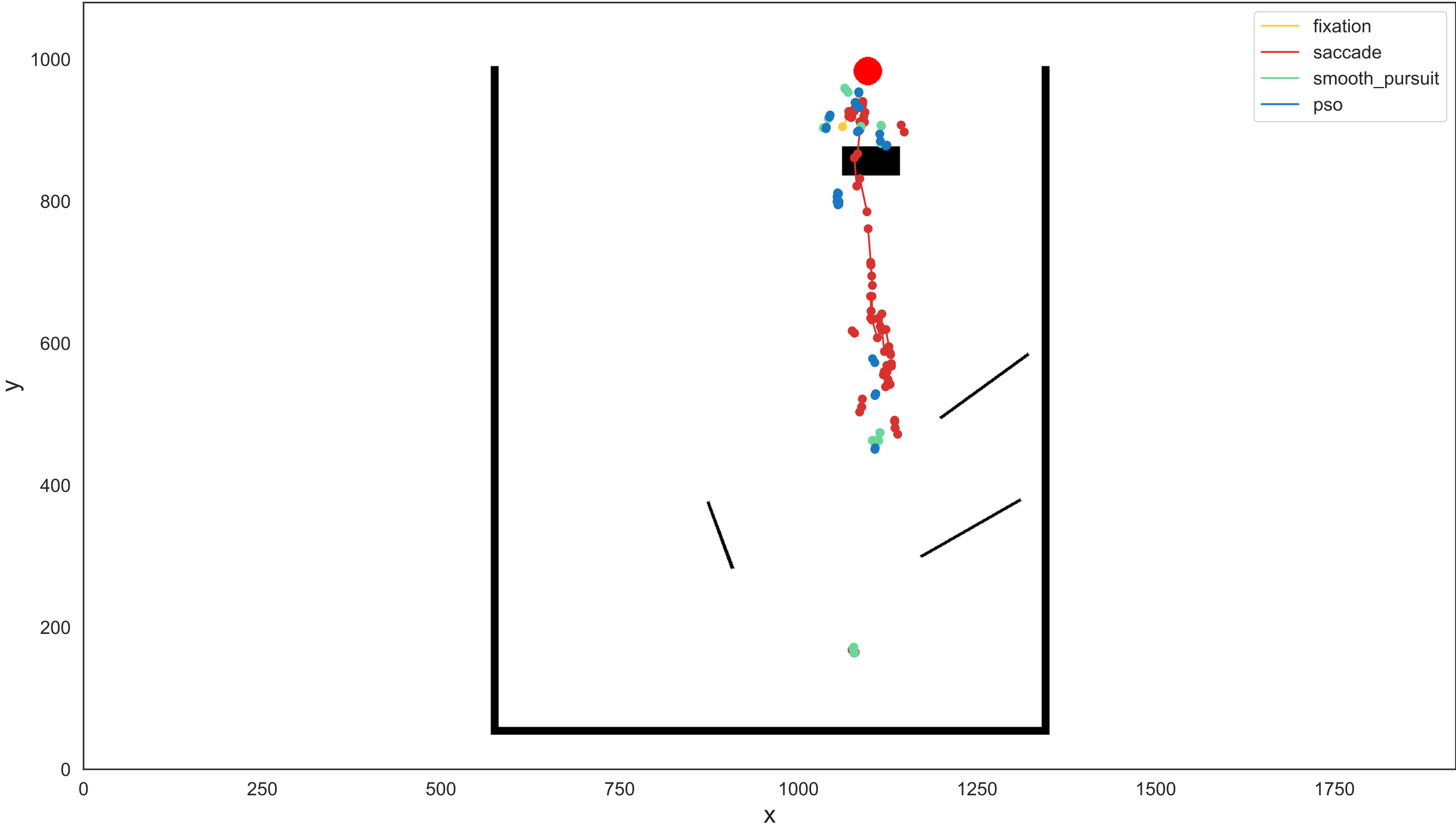
Scene: scene_2_1
