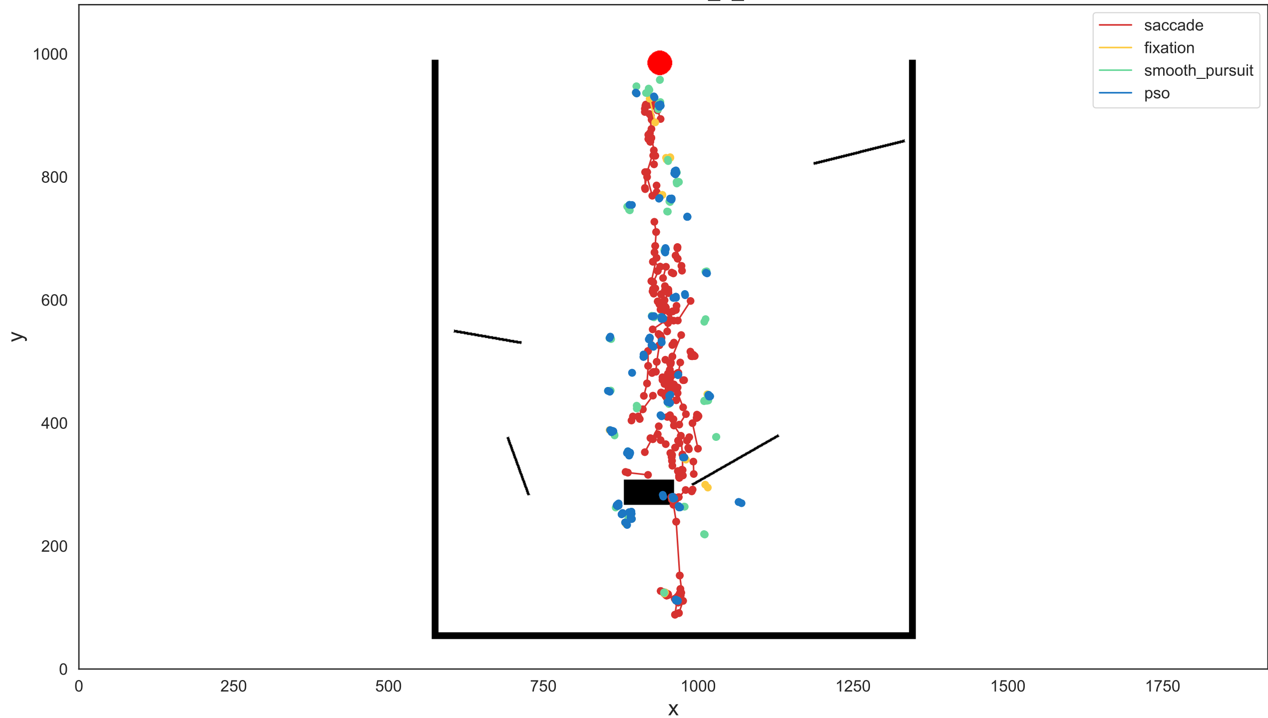
Scene: scene_2_23
