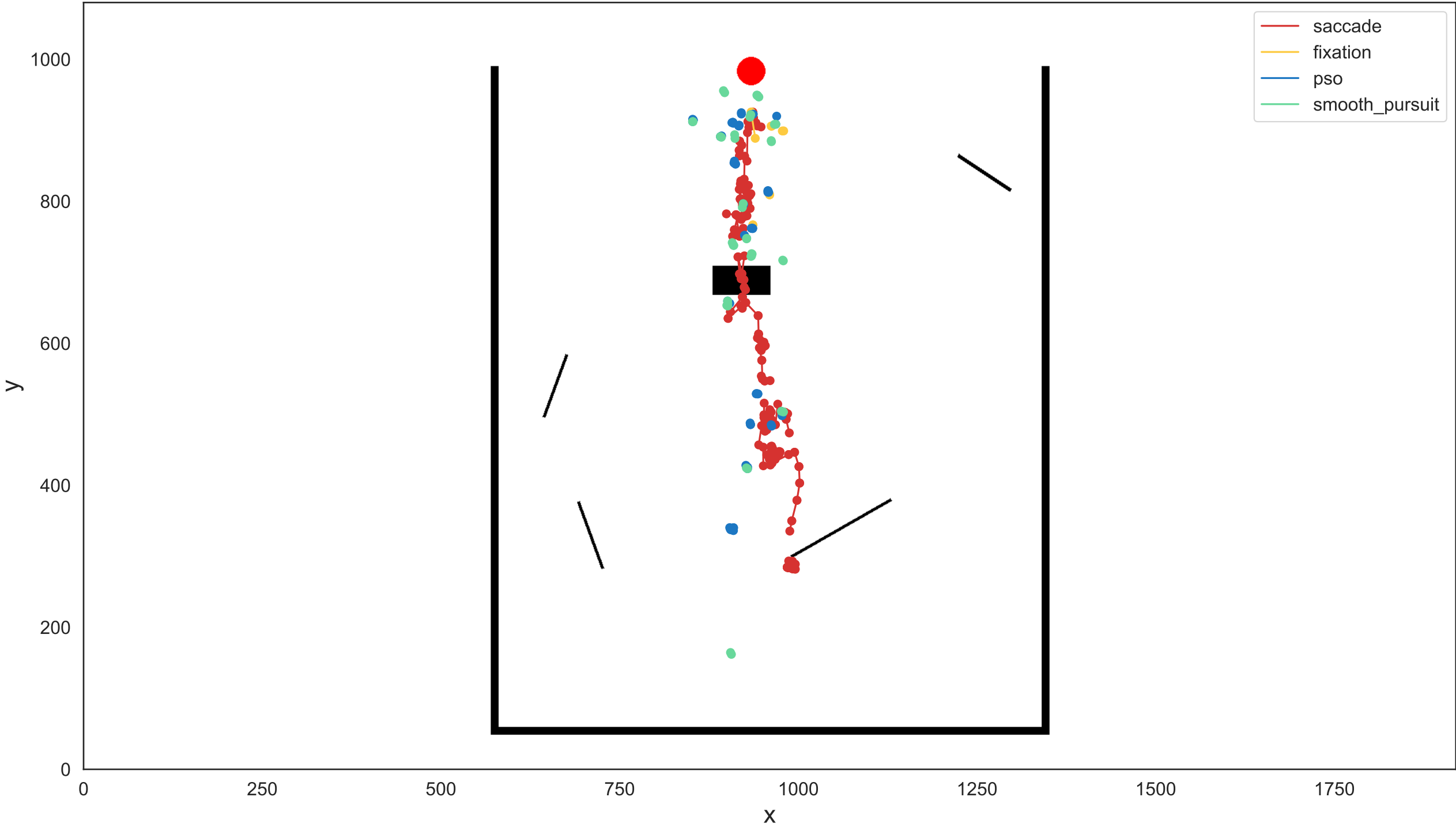
Scene: scene_2_9
