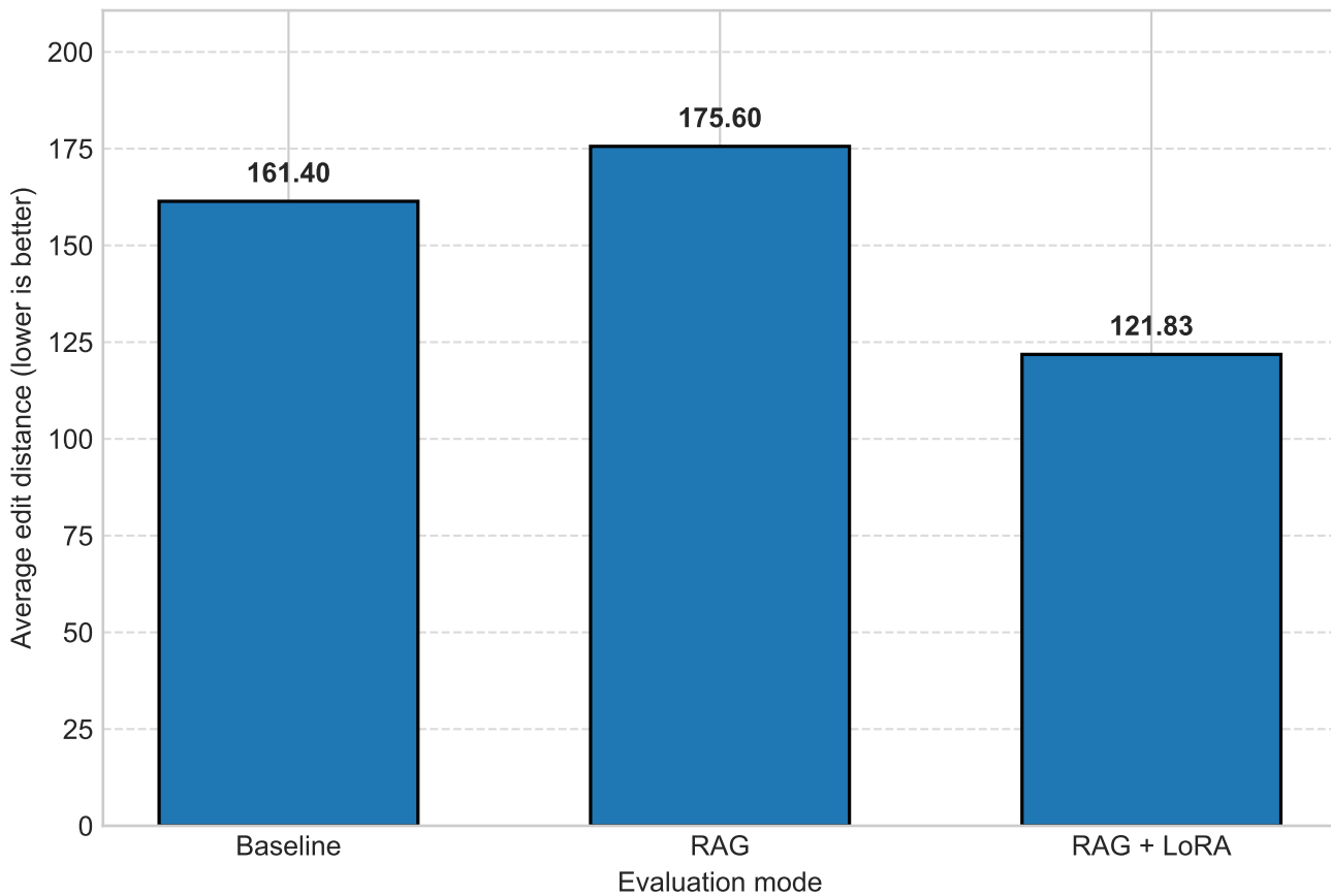
FIM Edit Distance – Gemma 2 2B-it
