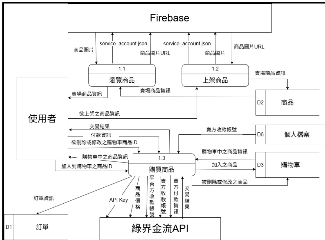
圖 12：DFD Level 2-1
