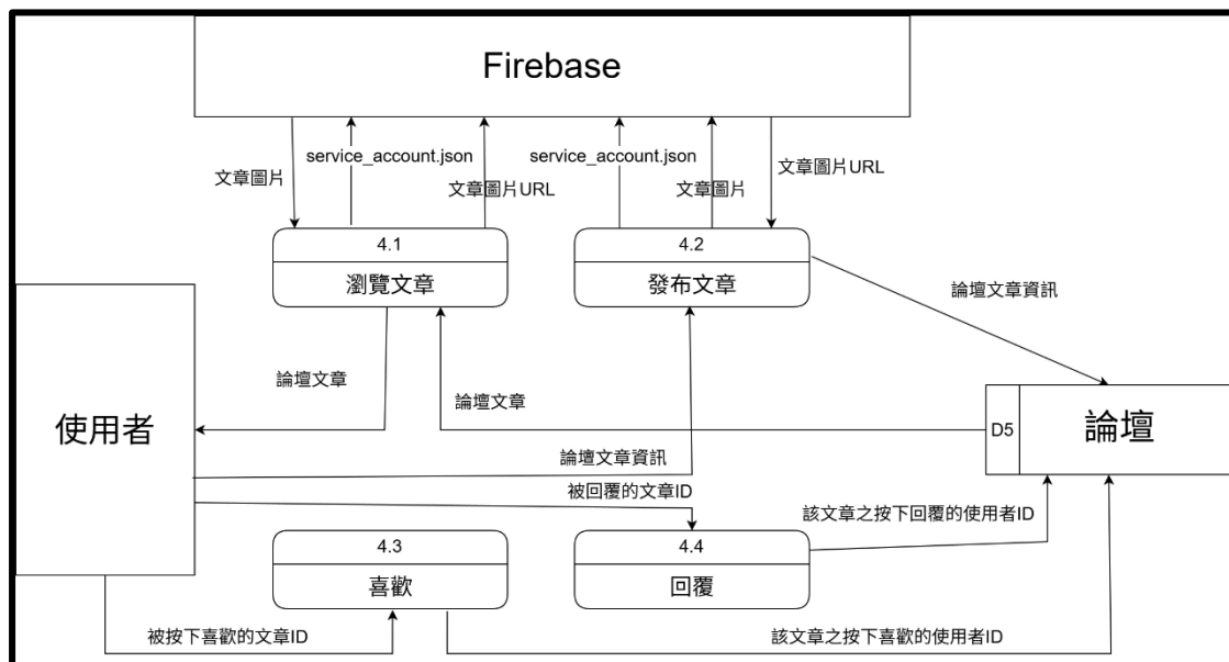
圖 13：DFD Level 2-2
