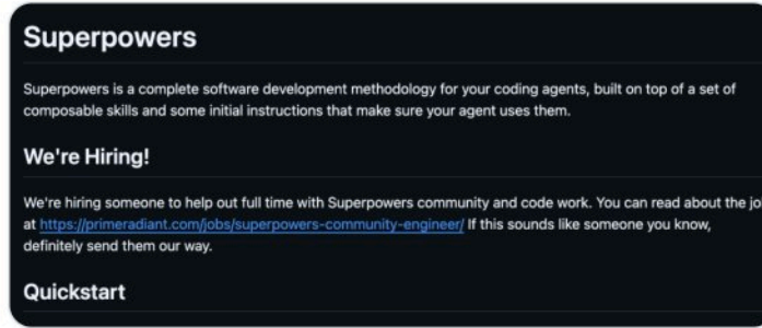
Superpowers
