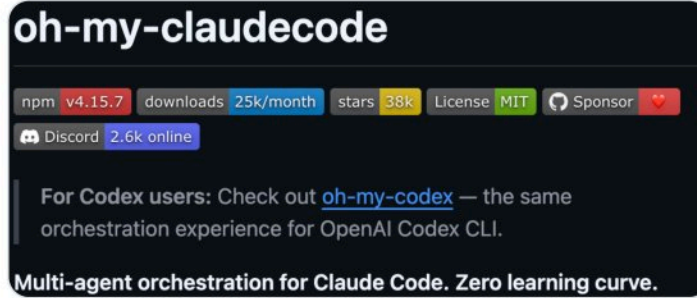
OMC 오마이클로드코드
