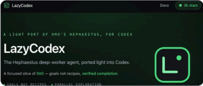
LazyCodex
