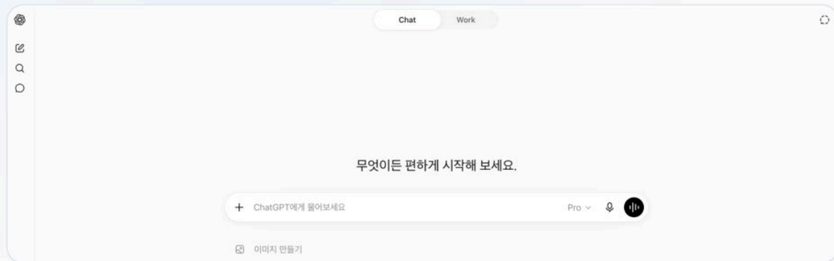
ChatGPT
