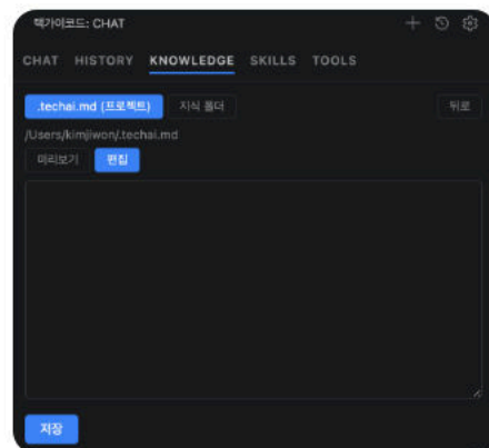
지식추가기능 · KNOWLEDGE
