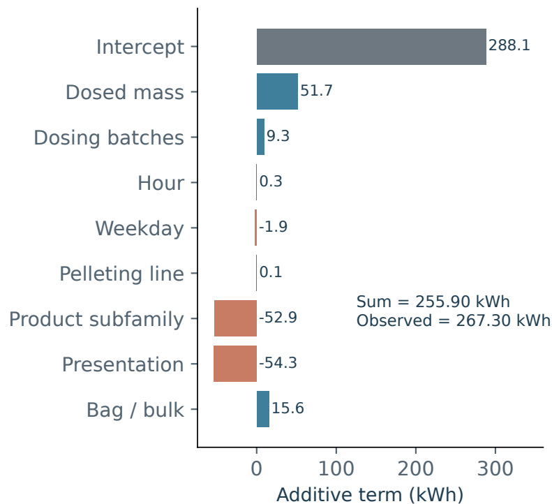
(d) Worked example: row 2080
