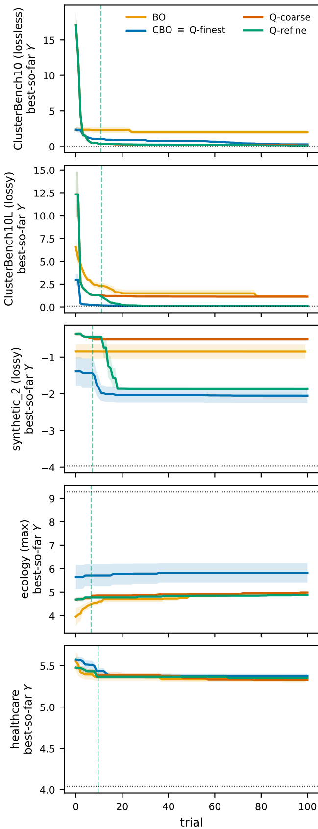
best-so-far Y
