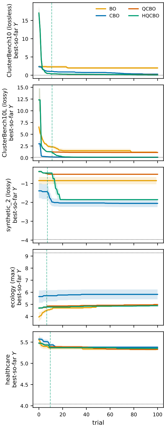
best-so-far Y
