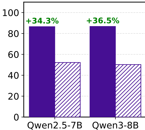
DP-Bird
