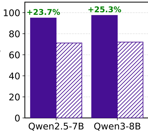
DP-Spider
