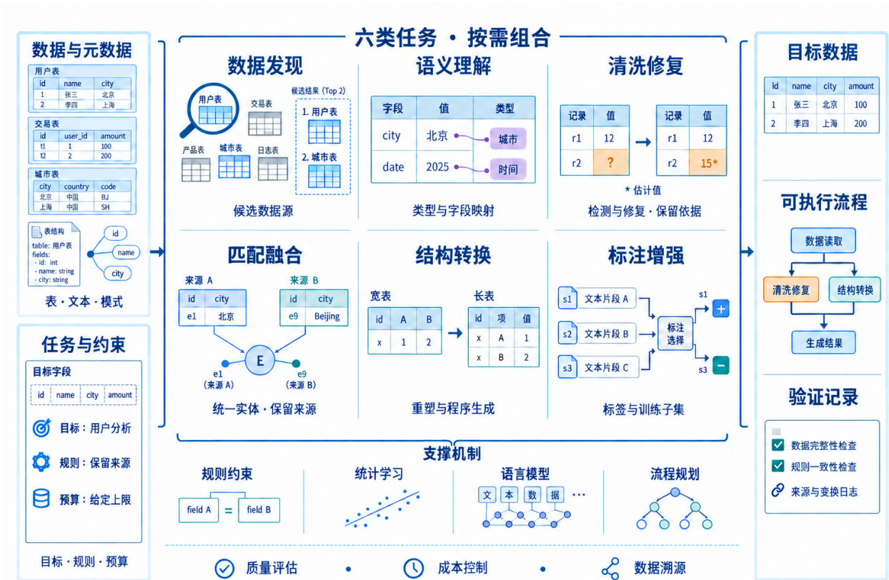
图 1 智能数据准备的任务体系。六类任务可根据下游目标组合, 规则约束、统计学习、语言模型与流程规划构成可互补的实现机制。局部数据用于机制示意, 星号表示估计值。图为本文综合归纳, 非特定系统架构。
