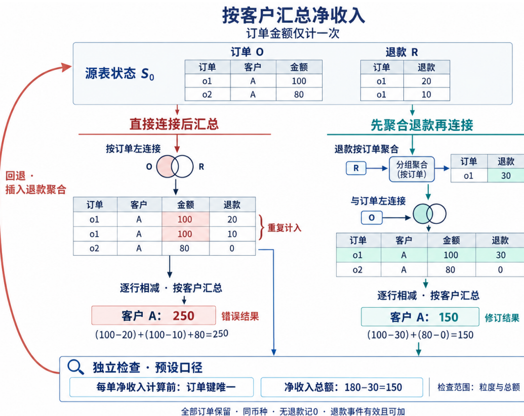
图 3 多表准备中粒度错误的传播、独立检查与回退。实例由本文构造; 250 与 150 是给定数据的确定性计算结果, 不是方法性能分数。检查依据来自预设任务口径。
