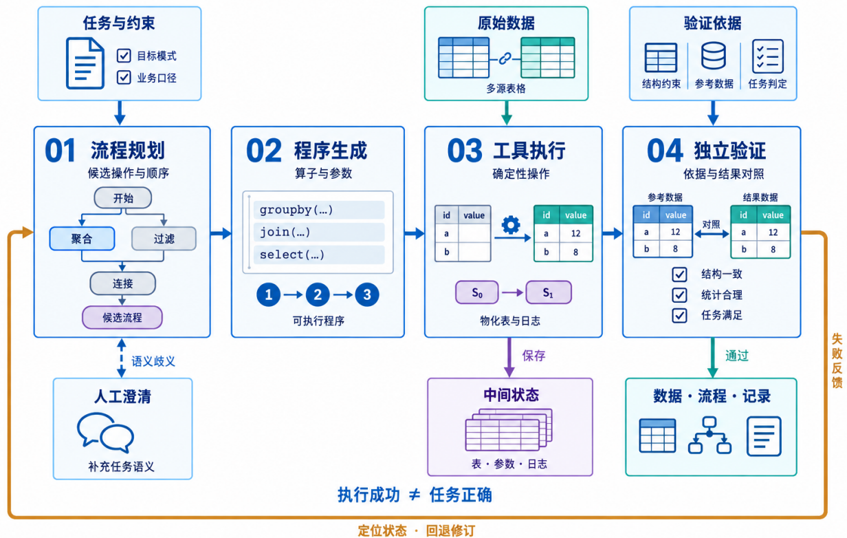
图 2 任务感知数据准备中的执行反馈与验证。实线表示主要处理及数据流，虚线表示语义澄清；验证失败后可定位中间状态并修订前序决策。微型表格与程序片段用于机制示意，该图不是 AutoPrep、DeepPrep 或 BAT 的原始架构图。
