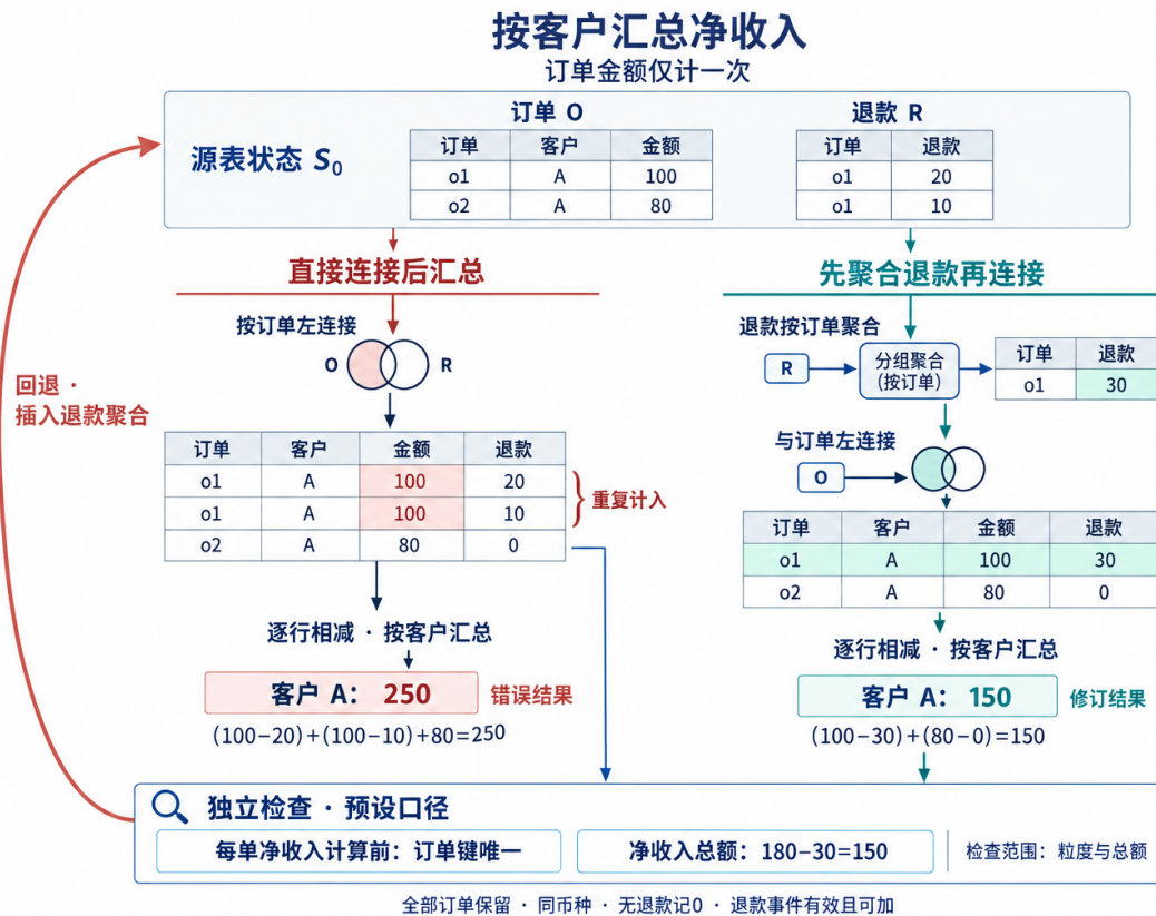
图 1 多表准备中粒度错误的传播、独立检查与回退。实例由本文构造; 250 与 150 是给定数据的确定性计算结果, 不是方法性能分数。检查依据来自预设任务口径。
