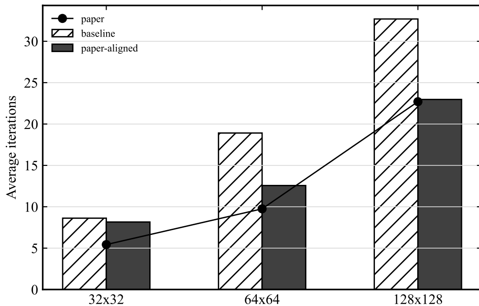
\eta = 0.50 , linear
