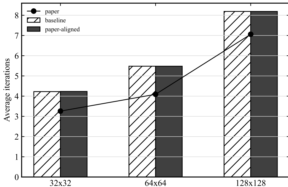
\eta = 0.50 , linear
