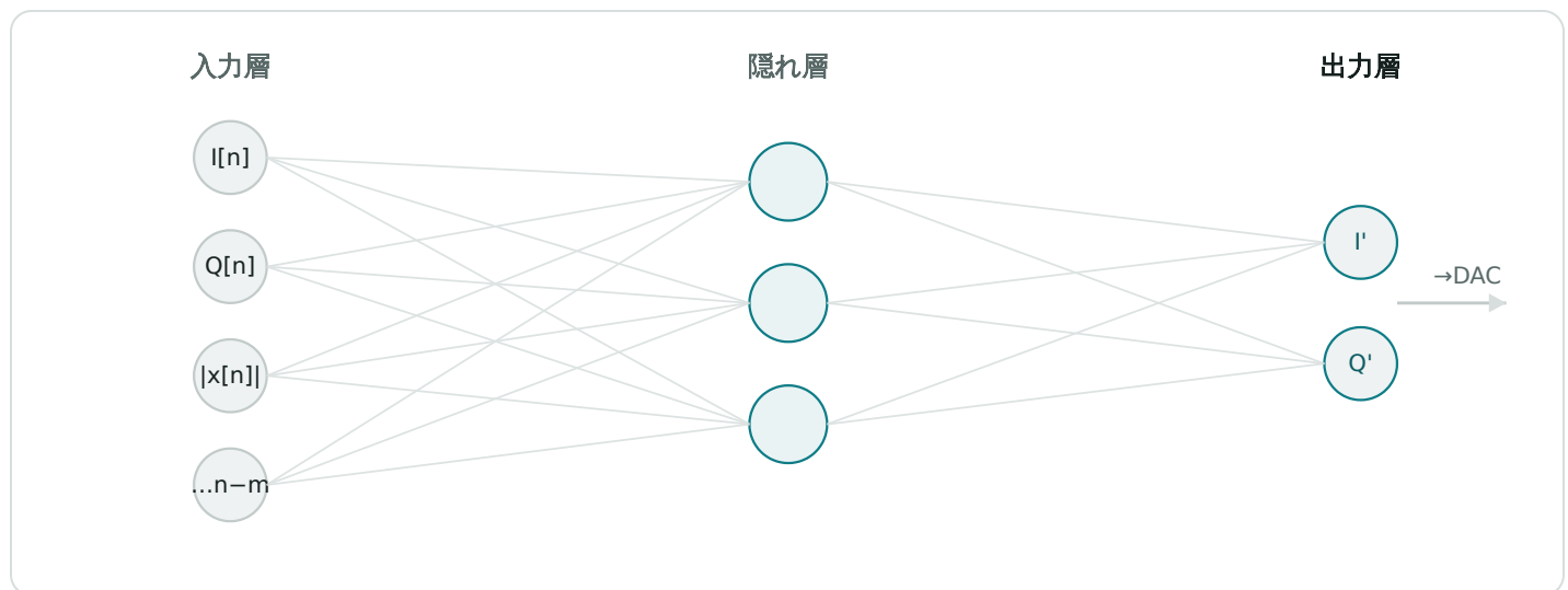
図 6.1 ニューラルネット DPD (実数値 MLP) の構造。現在・過去サンプルの I/Q と振幅特徴を入力にとり、隠れ層を経て予歪後の I/Q を出す。基底を人が設計する MP と違い、基底そのものを学習する。
