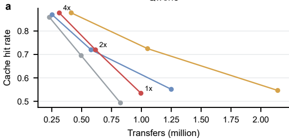
Qwen3
