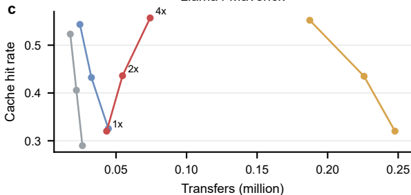
Llama4 Maverick
