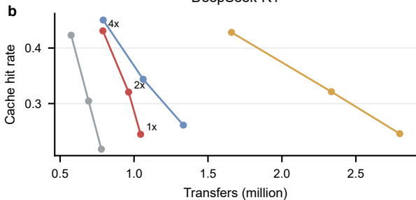
DeepSeek-R1
