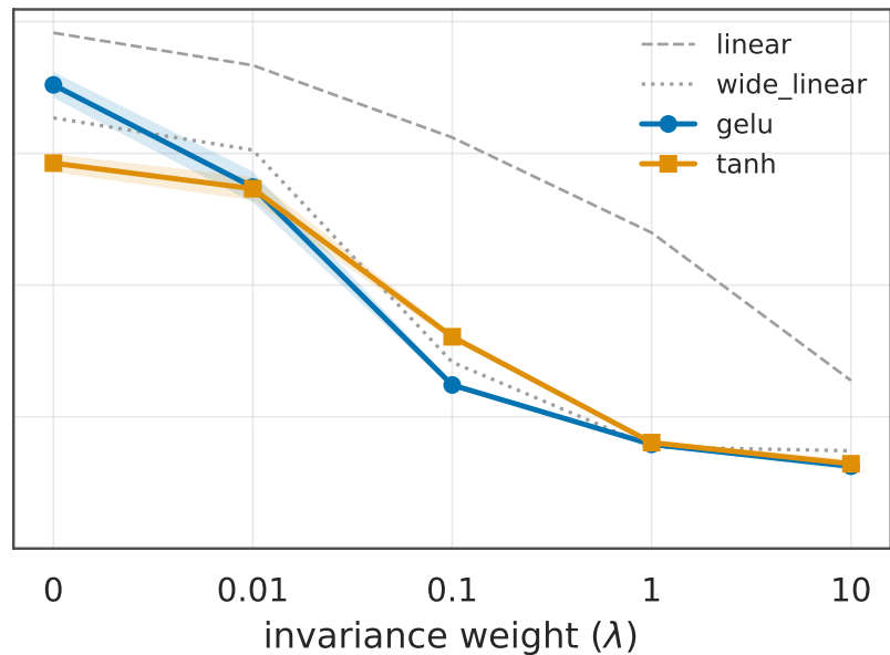
jina-v2
