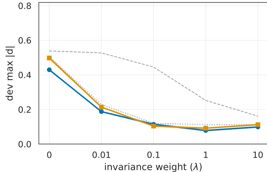
mxbai-v1
