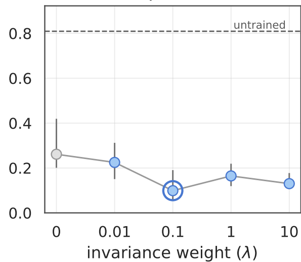
jina-v2
