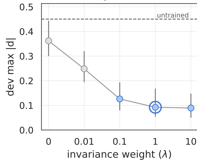
bge-v2-m3
