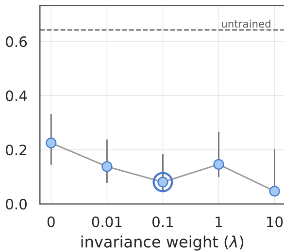
mxbai-v1
