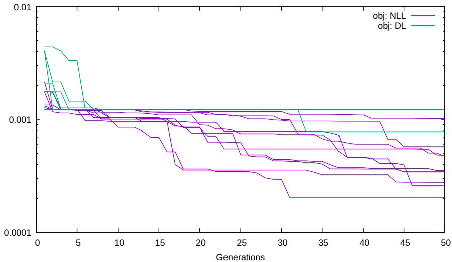
Nikuradse 1
