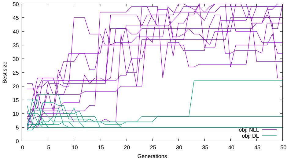
Nikuradse 1
