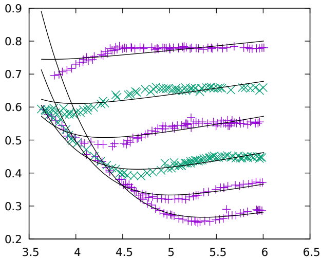
Nikuradse 1 Best NLL Solution
