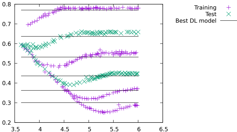
Nikuradse 1 Best DL Solution
