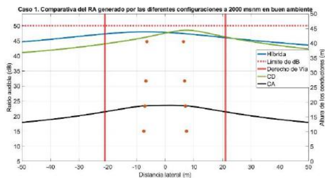
Figura 3.- Perfiles de RA en ambiente seco de la línea de México.
