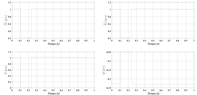
Figura 5.-Resultados de la simulación con el modelo REGC_A.
