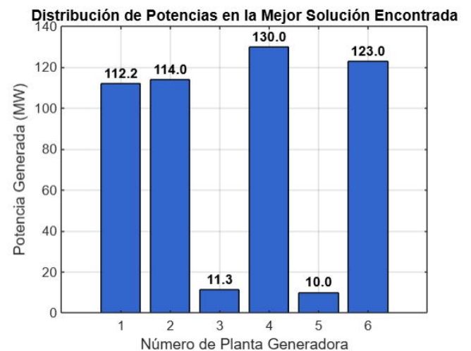
Figura 3.- Distribución de potencia de las plantas generadoras en la mejor solución encontrada.
