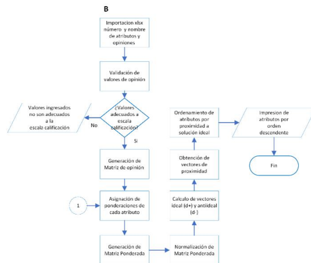
Figura 3.- Diagrama de flujo para la implementación del método TOPSIS en MATLAB.
