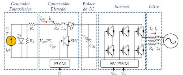
Figura 4.- Esquema de la planta solar fotovoltaica (Adaptada de [6]).
