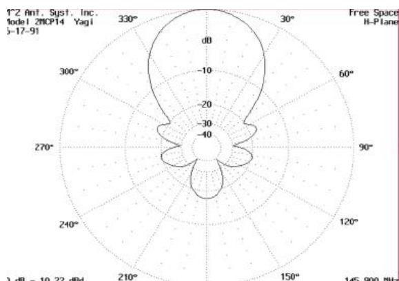
Figura 4 Patrón de radiación de antena
