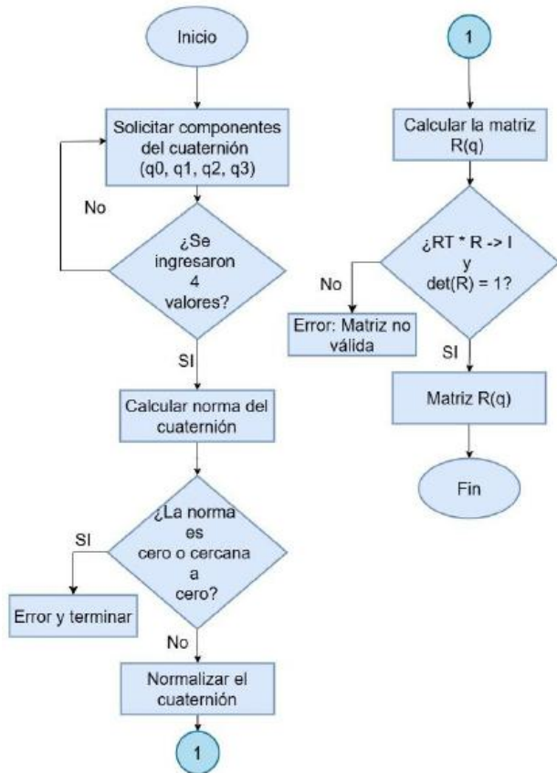
Figura. 1- Diagrama de flujo algoritmo construcción matriz de rotación cuaterniónica.
