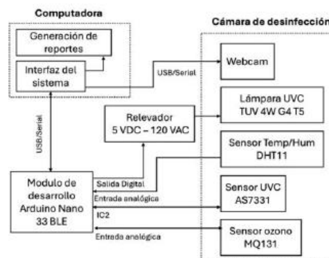
Figura 1.- Diagrama de bloques para desinfección de semillas.
