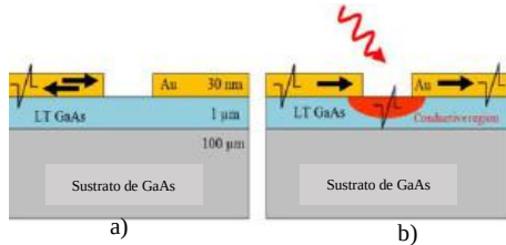
Figura 1.- Estado a) no conducción (OFF) y b) conducción ON [5].
