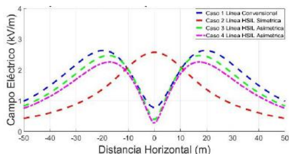
Figura 8.- Comparación de perfiles de campo eléctrico de los 4 casos.
