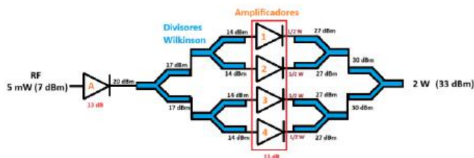
Figura 1. Imagen representativa del amplificador con redes Wilkinson.
