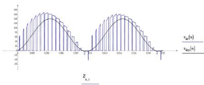
Figura 8.- Corriente directa consumida de la fuente de CD, en ambos modelos
