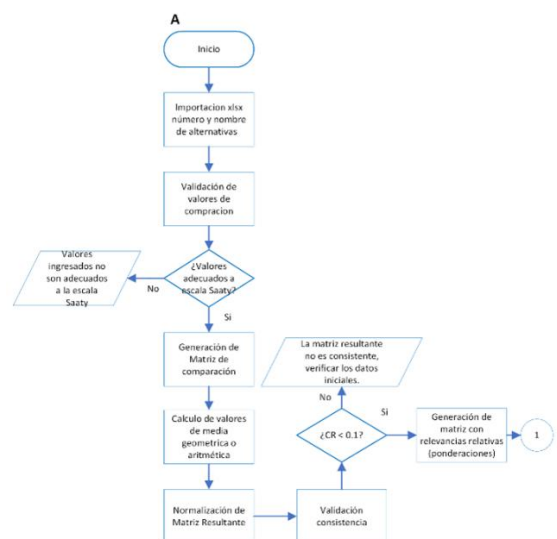
Figura 2.- Diagrama de flujo para la implementación del método AHP en MATLAB.
