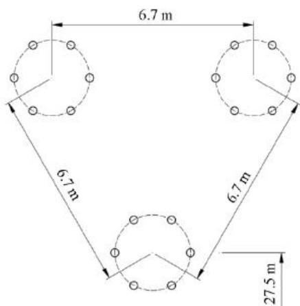
Figura 2.- Caso 2: línea de transmisión HSIL convencional con 6 conductores por fase.
