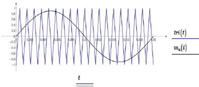
Figura 1.- Comparativa de señal senoidal y la portadora.
