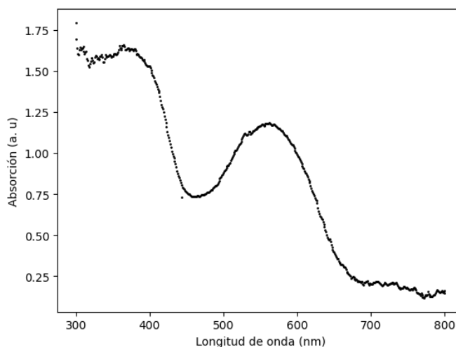
Figura 5.- Espectro de absorción óptica de la AC.
