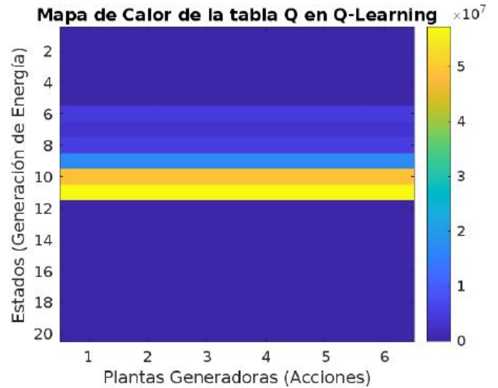
Figura 2.- Mapa de calor de la tabla Q después del entrenamiento.
