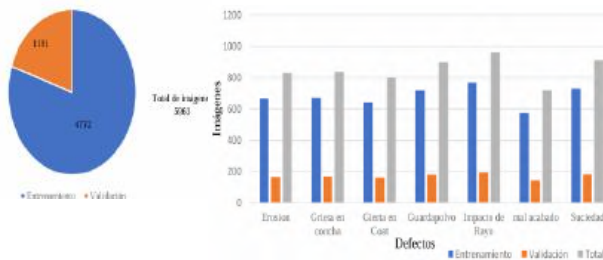
Figura 4.- Distribución de los defectos de los álaves siguiendo el criterio de Goodfellow.
