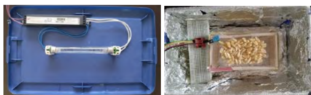
Figura 3.- Prototipo de cámara de desinfección.
