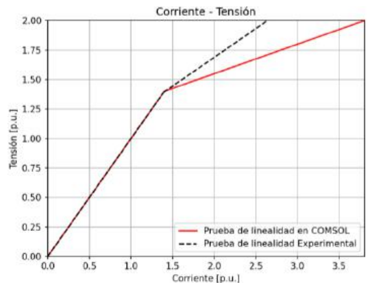
Figura 11. Comparación entre la curva obtenida con la prueba de linealidad y la curva obtenida con los resultados en COMSOL®
