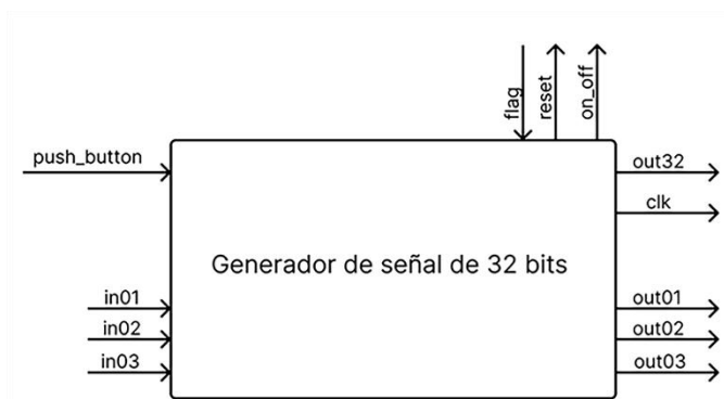
Figura 2. -Diagrama a bloques de generador de señal de 32 bits.
