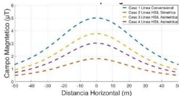
Figura 9.- Comparación de perfiles de campo magnético de los 4 casos.
