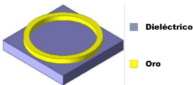
Figura 3. Representación gráfica de la celda unitaria propuesta en este trabajo para analizar el comportamiento de la SSF, donde el color azul corresponde al dieléctrico y el color amarillo a la geometría tipo anillo de oro.
