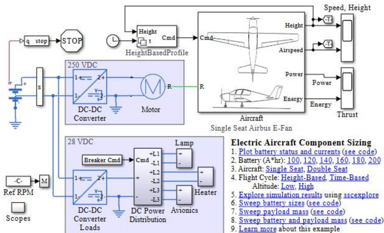
Figura 1. Modelo de una aeronave monoplaza [7].
