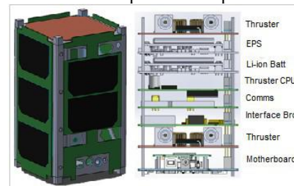
Figure 2: BRICSAT-2 (USNAPI) (NO-103).
