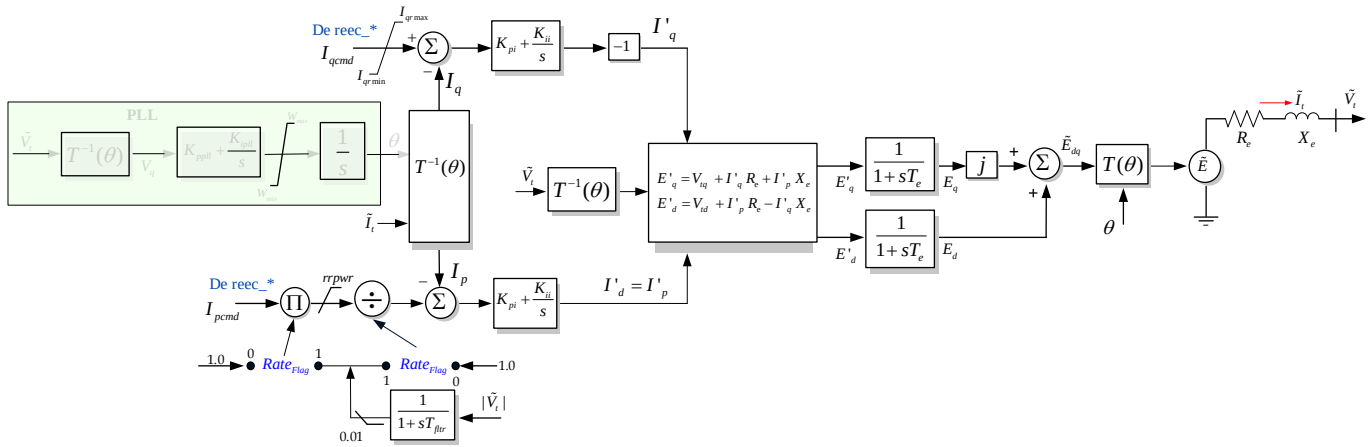
Figura 3.-Diagrama de bloques del modelo REGC_C.
