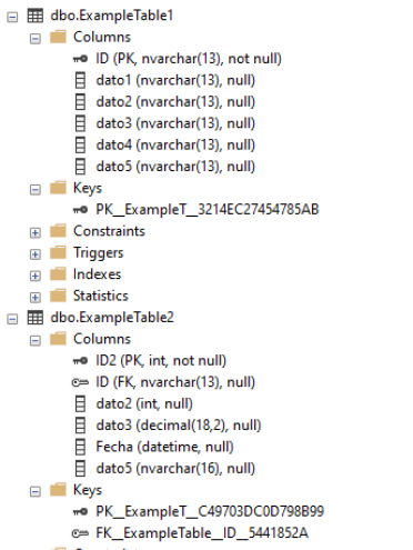
Figura 7.- Tabla generada en base de datos con llave primaria y asignacion de llave secundaria. Elaboración propia 2025
