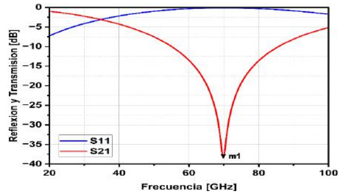
Figura 5. Reflexión y transmisión de la SSF utilizando como dielectrico el polimero polidimetilsiloxano (PDMS) y la geometria tipo anillo
