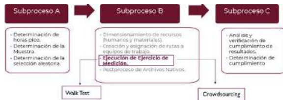
Figura 1.- Esquema de los subprocesos de la Metodología del IFT para evaluar la calidad de servicio de una red móvil de cobertura nacional.
