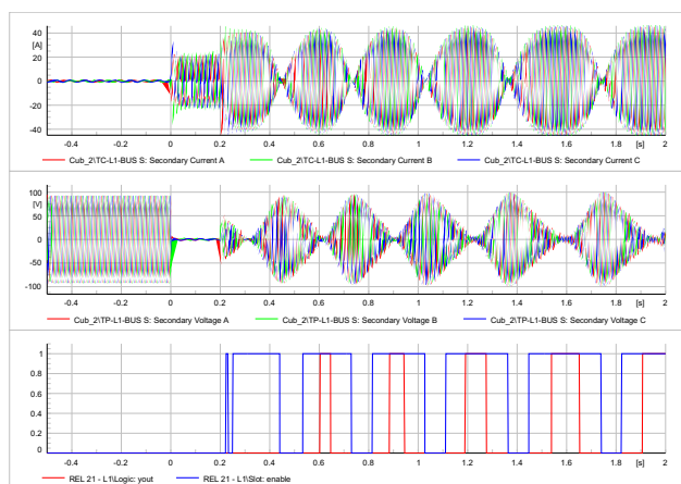
Figura 8.- Bloqueo por oscilación de potencia método convencional.
