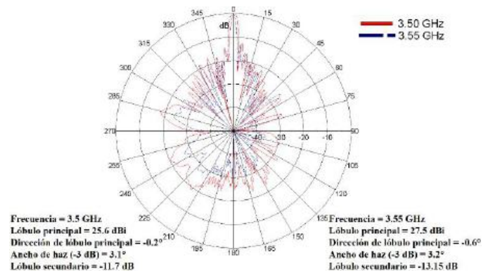
Figura 6.- Diagrama de radiación del arreglo de antenas construido caracterizado en 3.5 GHz y 3.55 GHz.
