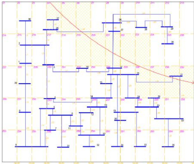
Figura 2. Trayectoria del huracán a través de la red IEEE-39.
