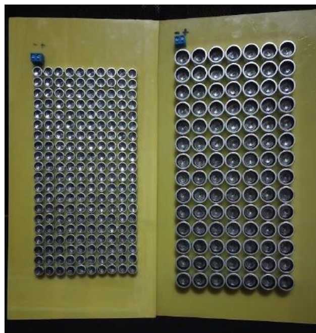
Figura 1.- Arreglos de transductores de alta frecuencia generados para la emisión de sonido direccionado.
