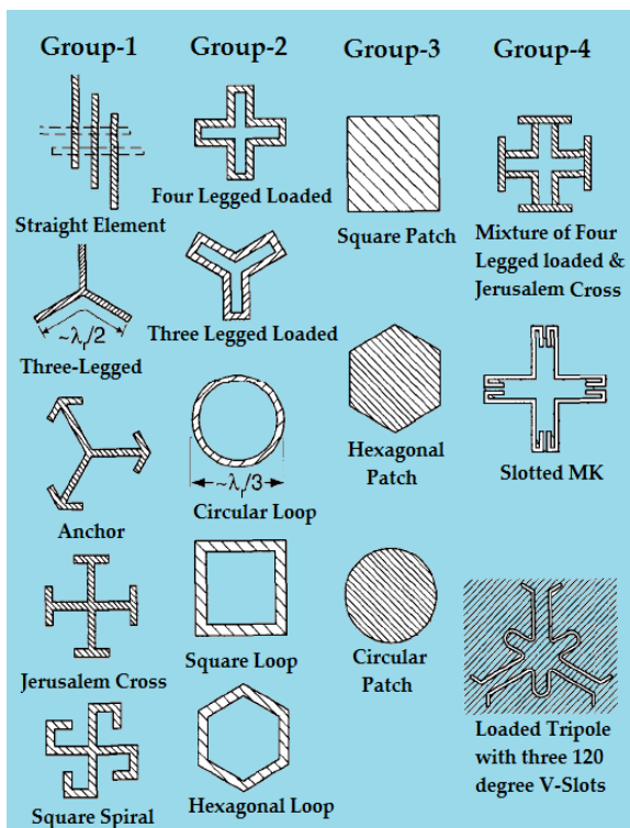
Figura 2. Clasificación y formas típicas de los elementos para SSF [2,15].
