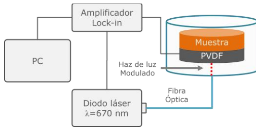
Figura 2.- Configuración experimental FPPE.
