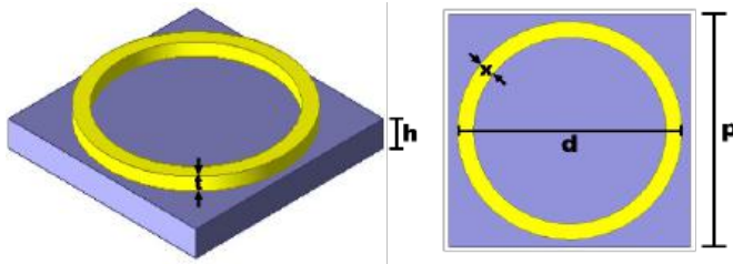
Figura 4. Parámetros de diseño para la SSF como los espesores ( h y t ), la periodicidad ( p ) y el diámetro del anillo( d ).
