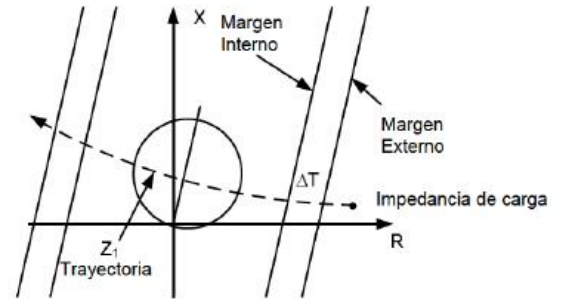
Figura 3.- Característica del margen de restricción doble (Dual-blinder characteristic).
