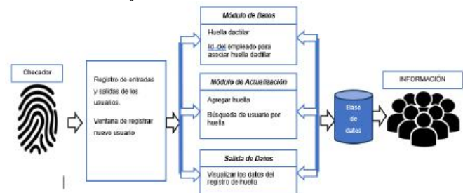
Figura 2.- Diseño de la arquitectura del sistema
