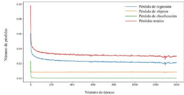
Figura 8.- Gráfica de pérdidas del entrenamiento.
