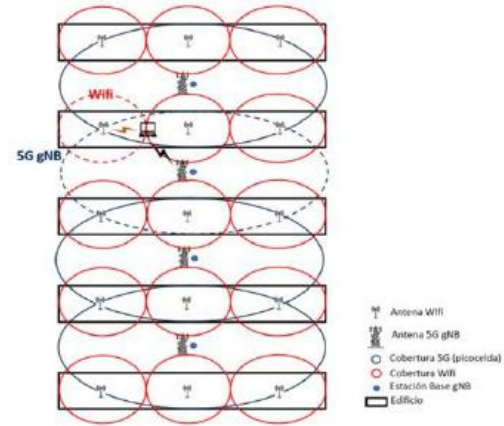
Figura 1.- Esquema de cobertura para ESIME unidad Zacatenco utilizando las RATs Wifi y 5G.
