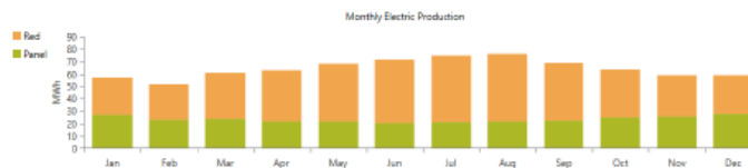
Figura 8.- Producción mensual del sistema
