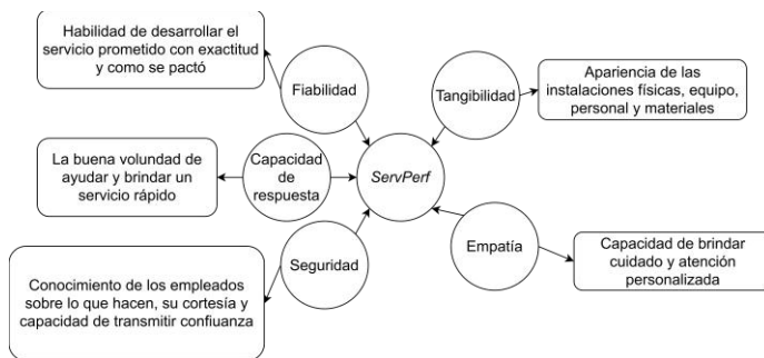
Figura1.- Modelo ServPerf .
