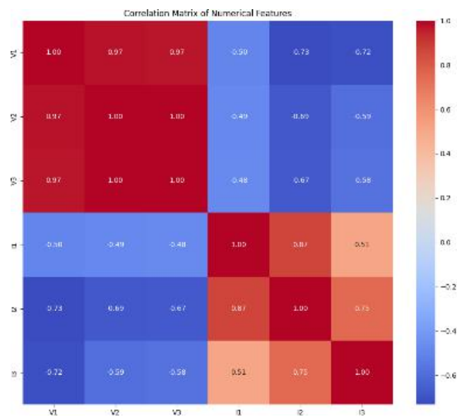
Figura 6.- Matriz de correlación
