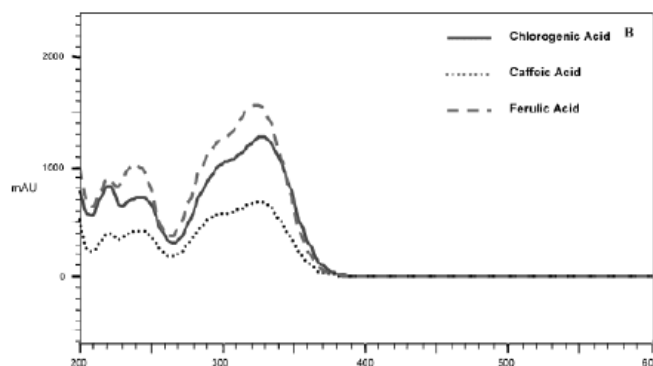
Figura 13.- Espectro de absorción de algunos tipos de ácidos fenólicos [18].
