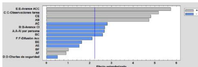
Figura 5.- Diagrama de Pareto Estandarizado para accidentes prevenidos por persona con interacciones de máximo orden de efecto 2 y exclusiones.
