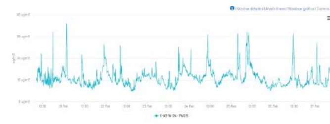
Figura 2: Comportamiento de PM 2.5 (obtenido de kunak cloud)
