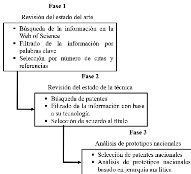
Figura 2. Metodología
