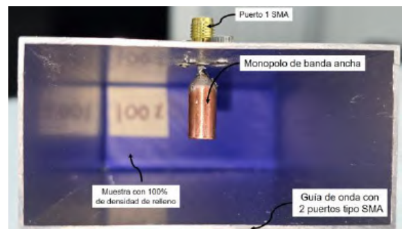
Figura 5.- Muestra dentro de la guía de onda.
