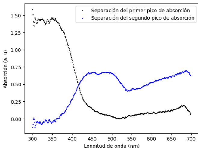
Figura 11.- Separación en la fase del espectro de absorción óptica de la SO.
