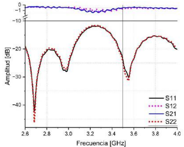
Figura 4.- Parámetros S medidos de la guía.
