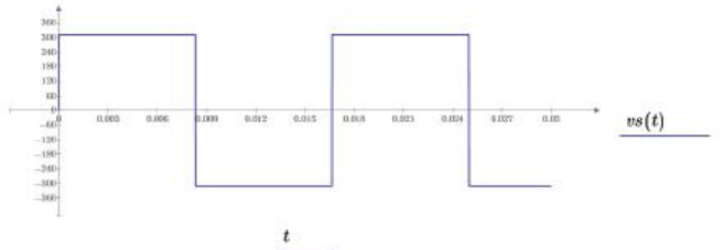
Figura 8.- Tensión de entrada de CA, onda cuadrada
