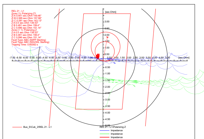
Figura 7.- Gráfica de la trayectoria de impedancia y características de los elementos de distancia y oscilación de potencia.
