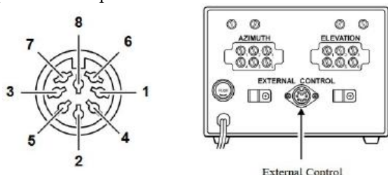
Figura 8 Puerto de control externo de los rotores
