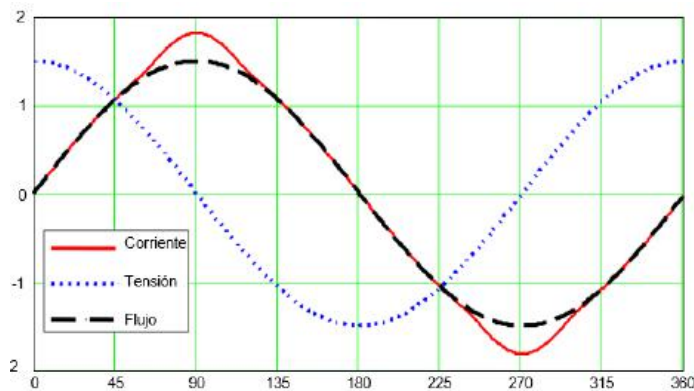
Figura 6. Ilustración de la forma de onda del flujo y corriente con una tensión sinusoidal aplicada a un inductor con una característica no lineal.
