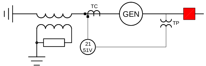
Figura 3.- Esquema de Protección de Respaldo del Generador.
