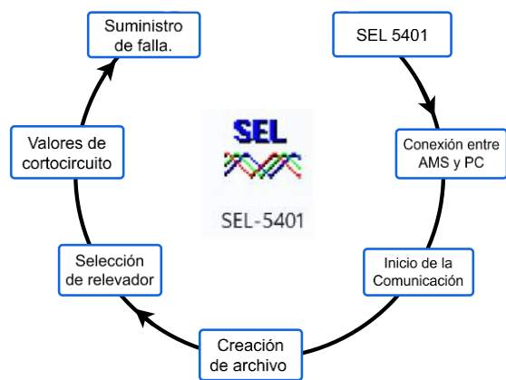
Figura 7.- Diagrama de bloques para suministrar la falla en los relés.
