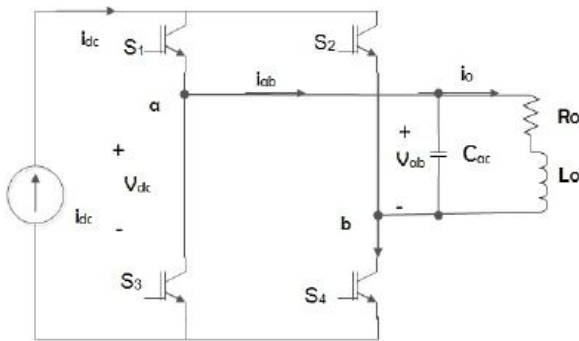
Figura 2.- Circuito equivalente inversor monofásico.
