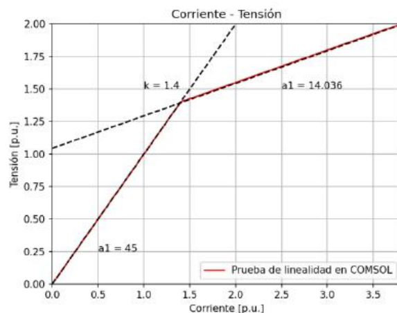
Figura 10. Curva de linealidad I-V calculada.
