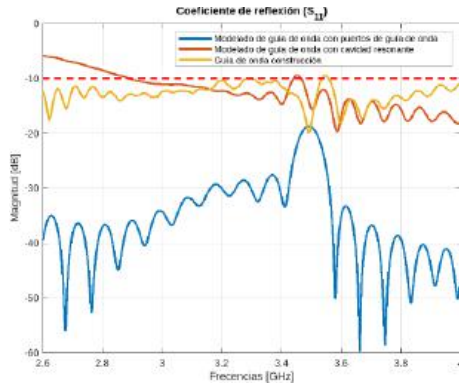
Figura 2.- Grafica comparativa entre el modelado contra lo construido.
