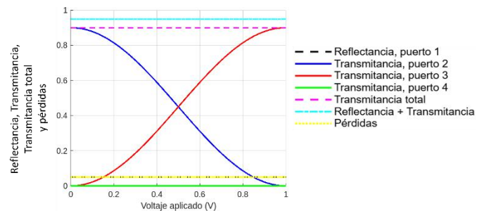
Figura 7.- Reflectancia, Transmitancia y Transmitancia total y pérdidas de un MZM de niobato de litio ( \text{LiNbO}_3 ).
