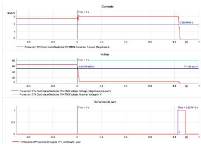
Figura 9.- Simulación dinámica de una Falla en Terminales del Transoformar Protección de Sobrecorriente Controlada por Voltaje.
