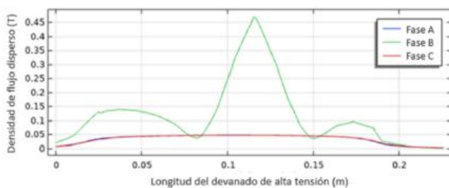
Figura 5.- Gráfica de la densidad de flujo disperso con falla en el devanado de alta tensión fase B.
