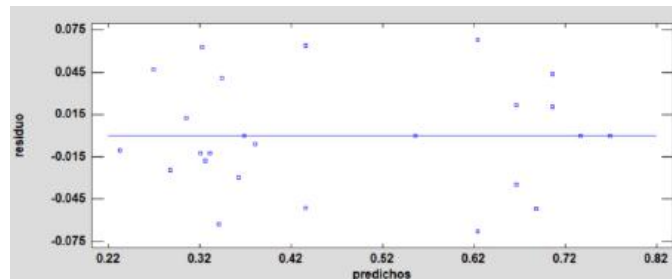
Figura 7.- Gráfico de residuos para accidentes por persona.
