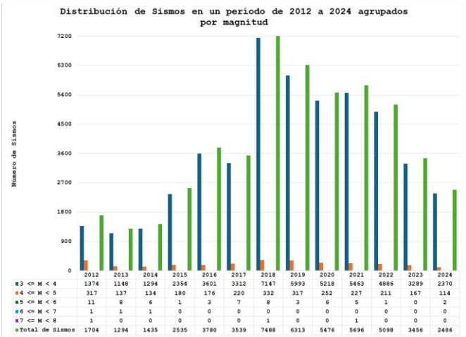
Figura 6. Distribución de Sismos en un periodo de 2012 a 2024 agrupados por magnitud.
