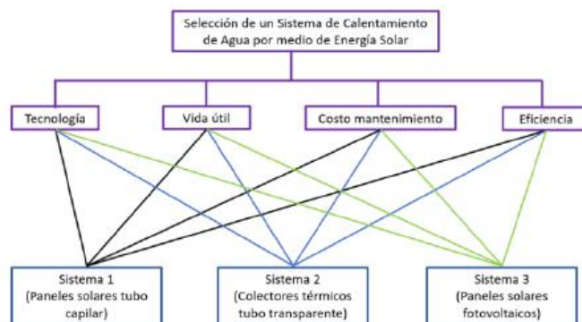
Figura 4.- Modelo Jerárquico
