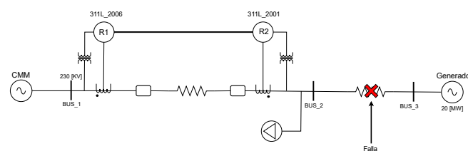
Figura 4.- Falla fuera de la zona de protección
