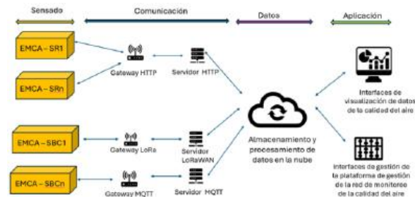
Figura 1: Estación de Monitoreo con Sensores Regulatorios y Sensores de Bajo Costo (Autoría propia).
