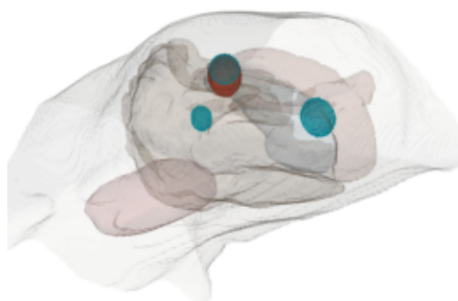
(d) Hard three-foci case 3 foci | ellipsoid + sphere
