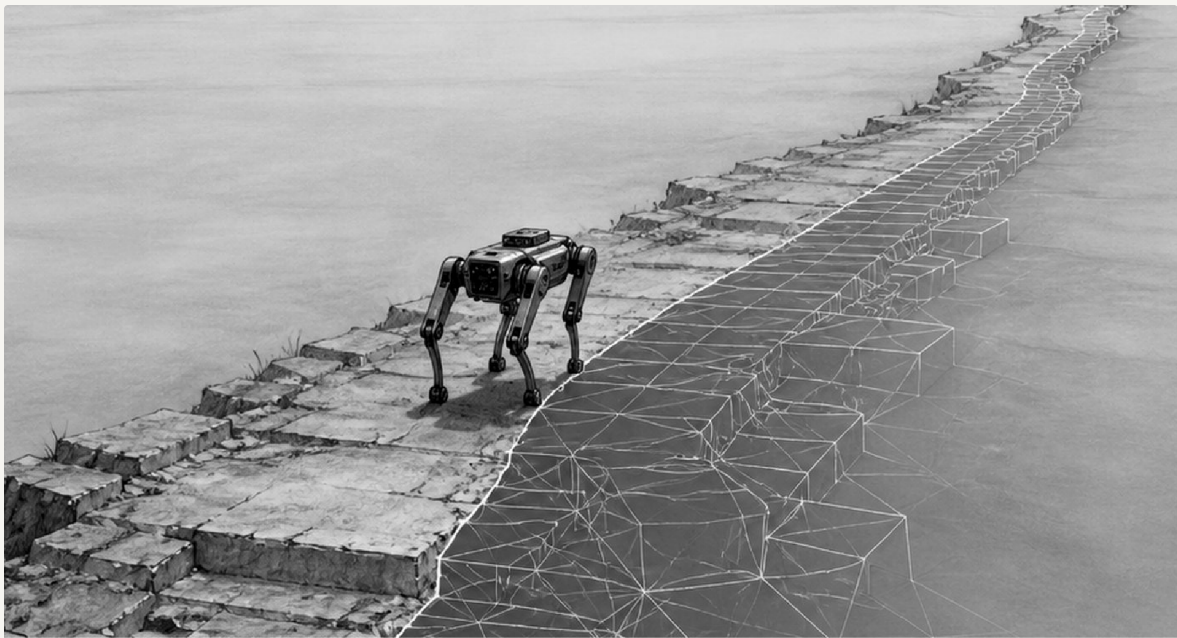
한 길인데 왼쪽은 실제 지면, 오른쪽은 시뮬레이션이 읽은 같은 지면
