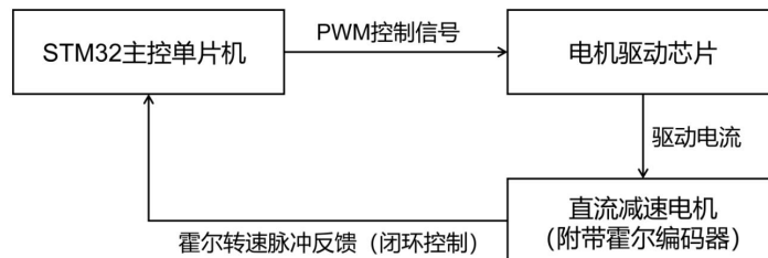
图 5 运动底盘控制系统连接图
