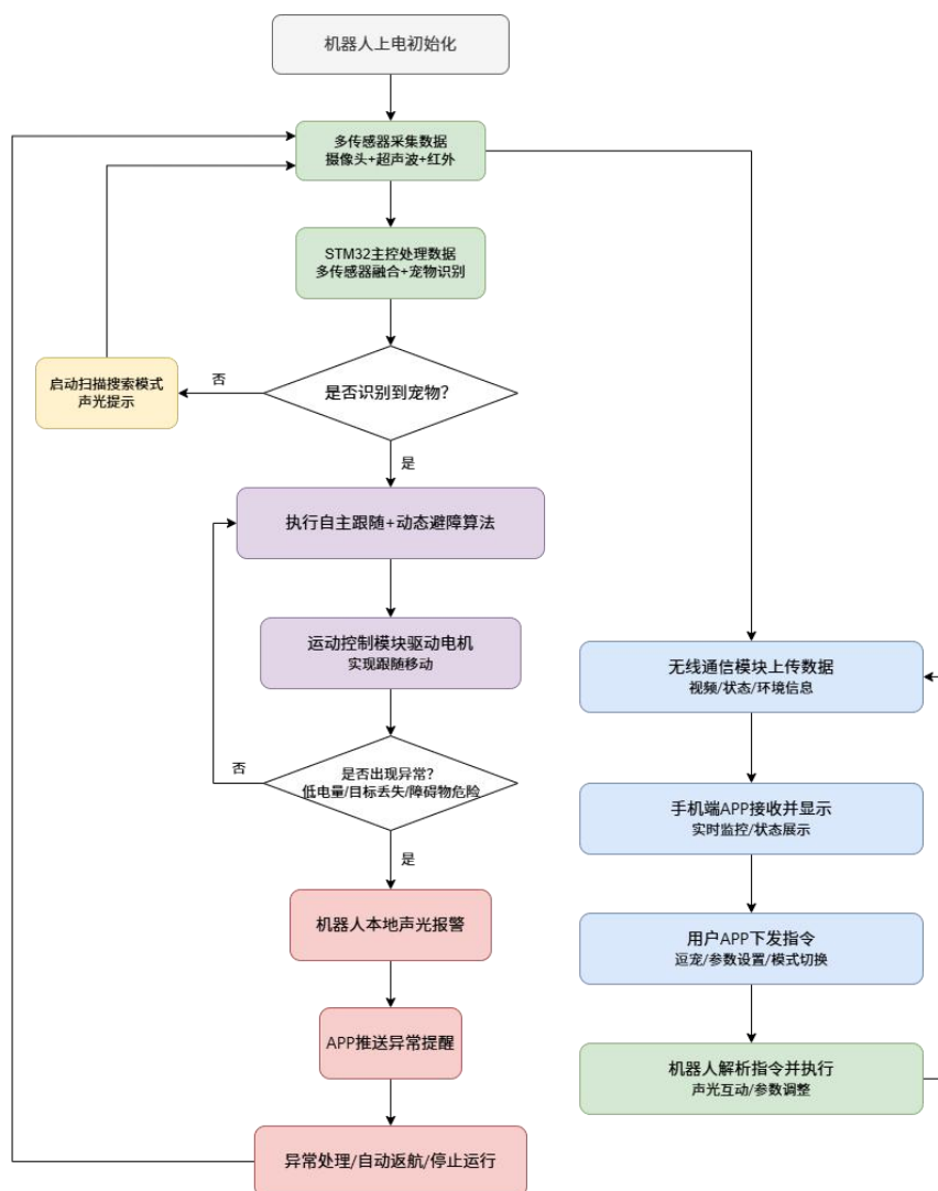
图 3 系统工作流程图
