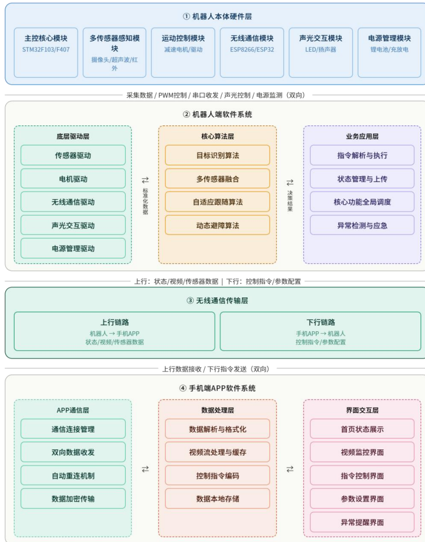
图 6 软件架构
