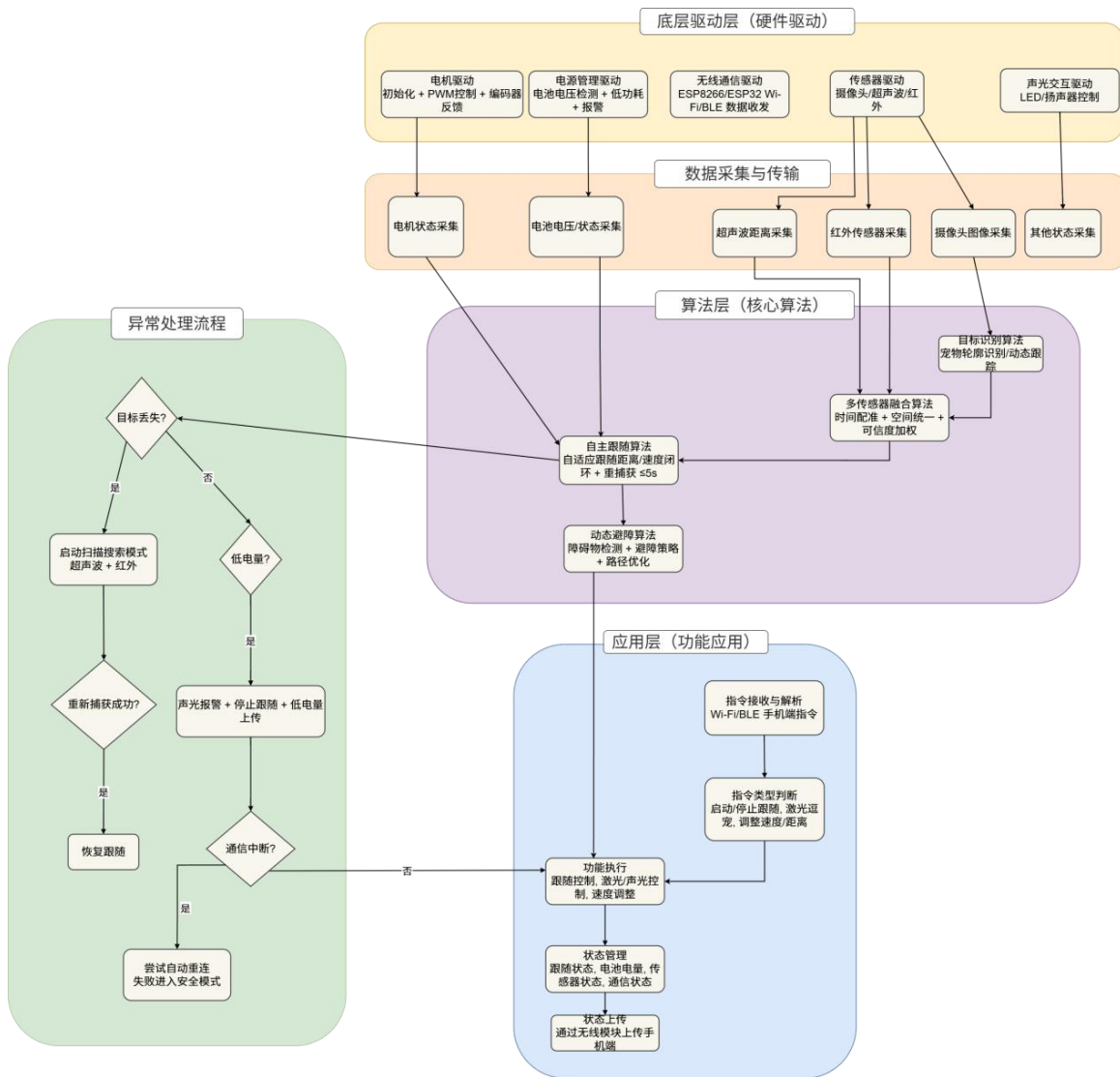
图 7 机器人端软件流程图
