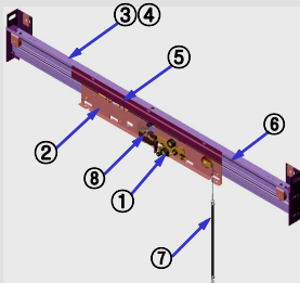
Door Rail
