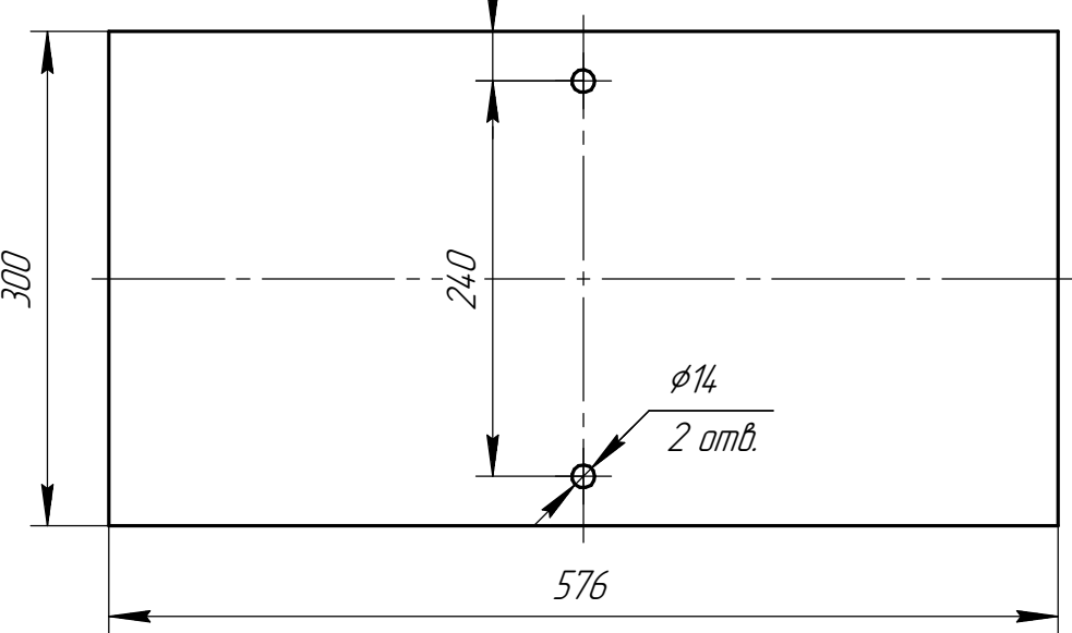
Дет. поз. 2 (1:1)
