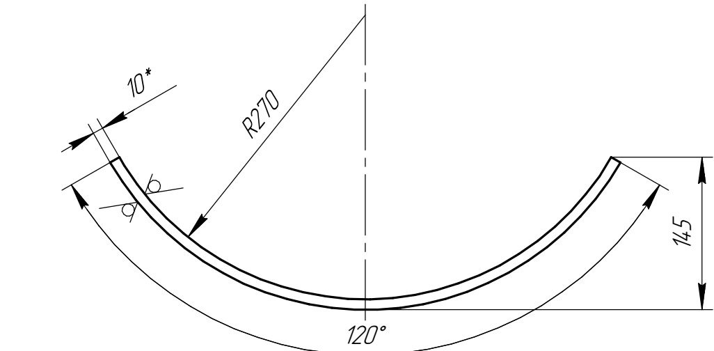
Дет. поз. 1 (1:5)
