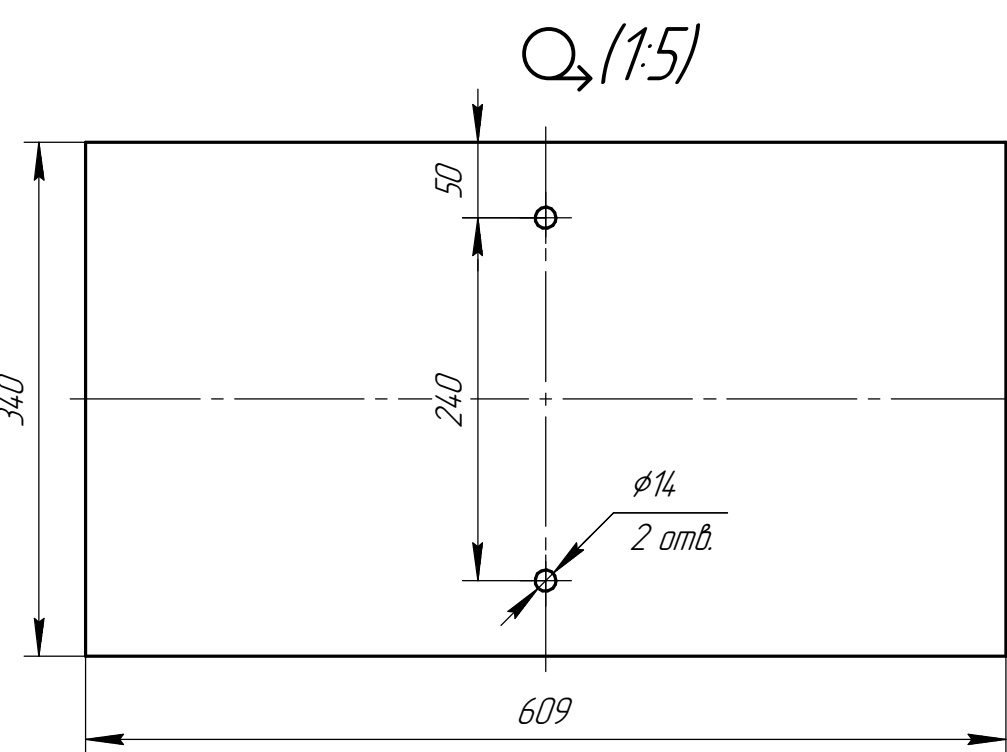
Дет. поз. 3
