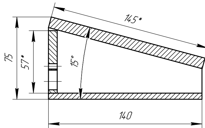
Дет. поз. 7 (1:5)
