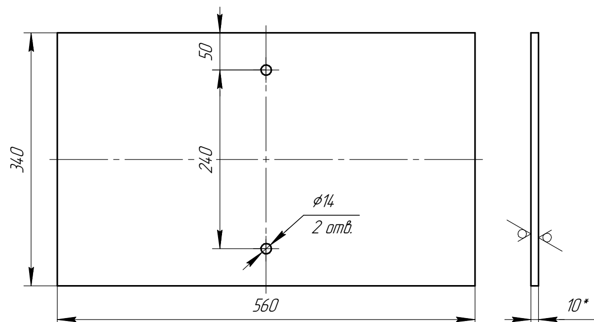
Дет. поз. 7.1 (1:5)
