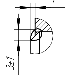
Дет. поз. 8.1 (1:1)
