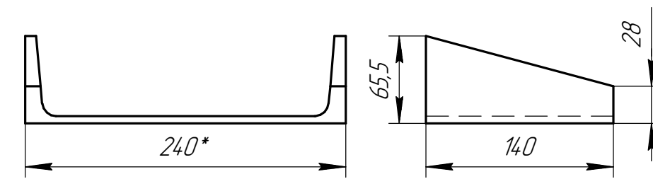
Дет. поз. 4.2
