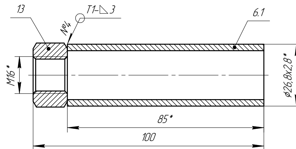
Дет. поз. 6 (1:1)
