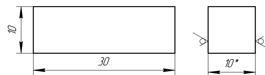
Дет. поз. 9 (2:1)
