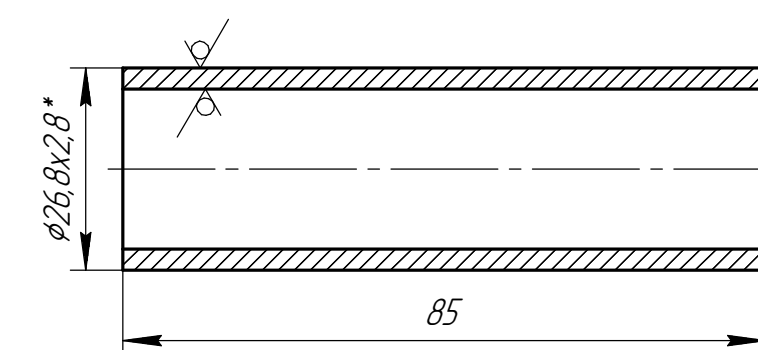
Дет. поз. 6.1 (1:1)
