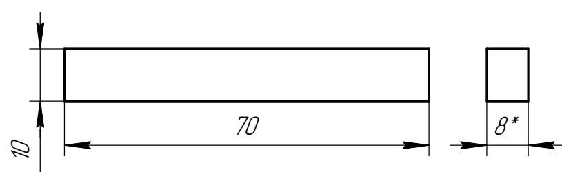
Дет. поз. 7.2 (1:1)
