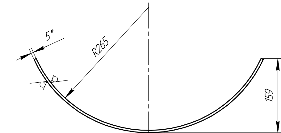
Дет. поз. 11 (1:5)
