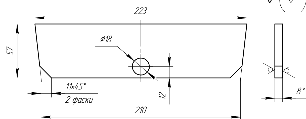
Дет. поз. 5.1 (1:2)
