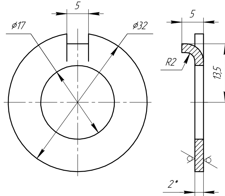
Дет. поз. 10 (2:1)
