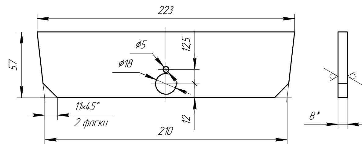
Дет. поз. 4.2
