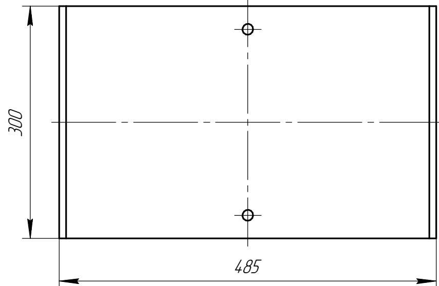
Дет. поз. 2 (1:1)
